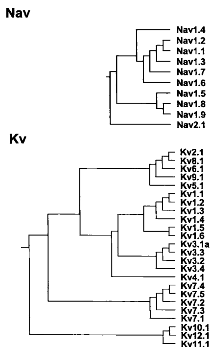
図2. 膜電位依存性Na + チャネル(Nav)とK + チャネル(Kv)のポアを形成する \alpha サブユニットの分子進化系統樹。近隣接合法(Neighbour-joining method)による。K + チャネルの系統樹は、代表的なものに限って作成してある。
