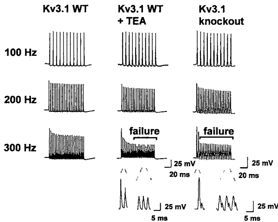
図6. 膜電位依存性 K^+ チャンネル Kv3.1 による聴神経核ニューロンの興奮調節. 電気刺激の頻度を増加してゆくと, Kv3.1 遺伝子をノックアウト (knockout) したマウス由来の内側台形体核 (MNTB) ニューロンの活動電位の振幅は, 野生型 (WT) マウス由来のMNTBニューロンに比べて著明に低下する (failure). K^+ チャンネル阻害薬のテトラエチルアンモニウム (TEA) の存在下の野生型MNTBニューロンでも同様である. 文献6より改変.
