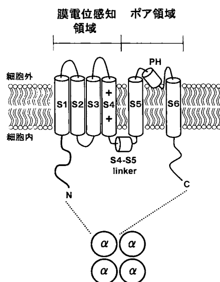
図1. 膜電位依存性 \text{K}^+ チャネルの \alpha サブユニットの基本構造。 \text{K}^+ チャネルは4量体の中央がイオンの通過路になる。 \text{Na}^+ チャネルの \alpha サブユニットと \text{Ca}^{2+} チャネルの \alpha_1 サブユニットでは, この基本単位が一本の長いペプチド内で4回繰り返してあり, これがイオンの通過路を囲む。
