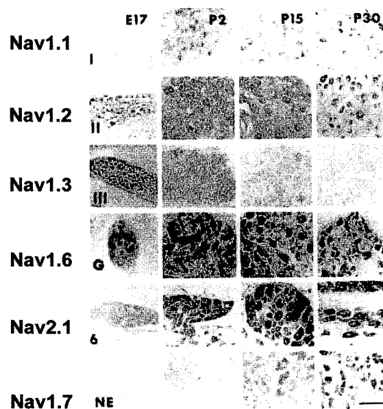
図3. 膜電位依存性Na + チャネル \alpha サブユニットの発達に伴う発現変化。ラット脊髄後根神経節に発現するNa + チャネルの \alpha サブユニットのmRNAを in situ ハイブリダイゼーション法にて検出。胎生17日(E17), 生後2, 15, 30日(P2, P15, P30)の組織を使用。文献4より改変。
