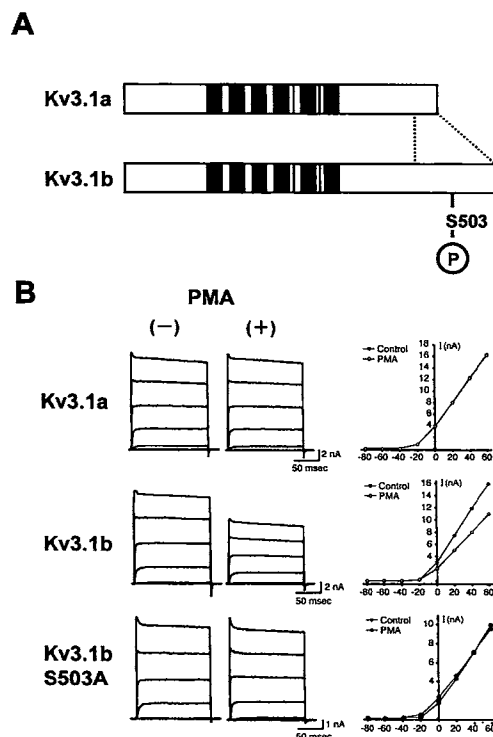
図5. 膜電位依存性K + チャネルKv3.1のC-キナーゼによる活動調節。A. 選択的スプライシングによって、C末端の異なるタンパク(Kv3.1aとKv3.1b)がつけられる。B. Kv3.1bの503番目のセリン残基(S503)をアラニン残基に置換すると、C-キナーゼの活性化剤であるホルボール12-ミリスチン酸13-酢酸(PMA)による電流抑制が観られなくなる。文献6より改変。
