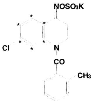
図1 [^{14}\text{C}]\text{M17055} の化学構造式 (*標識部位)
