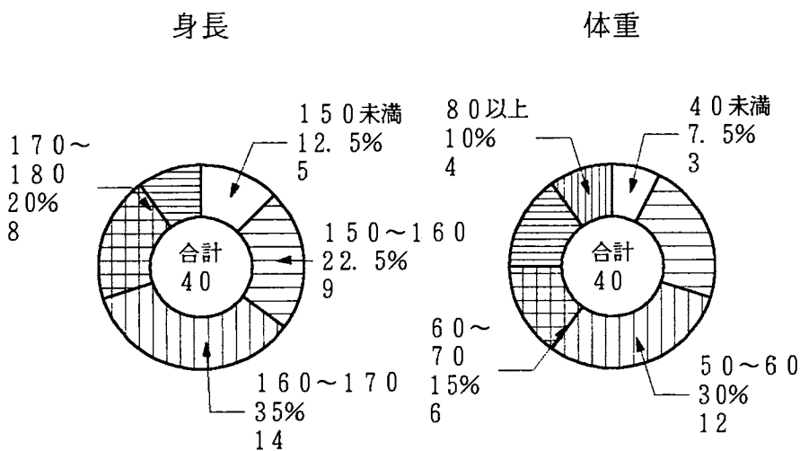
図2. 7 出力結果
