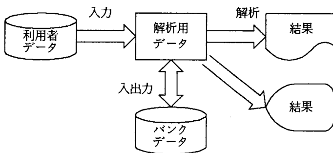
図1. 4 実行の流れ
