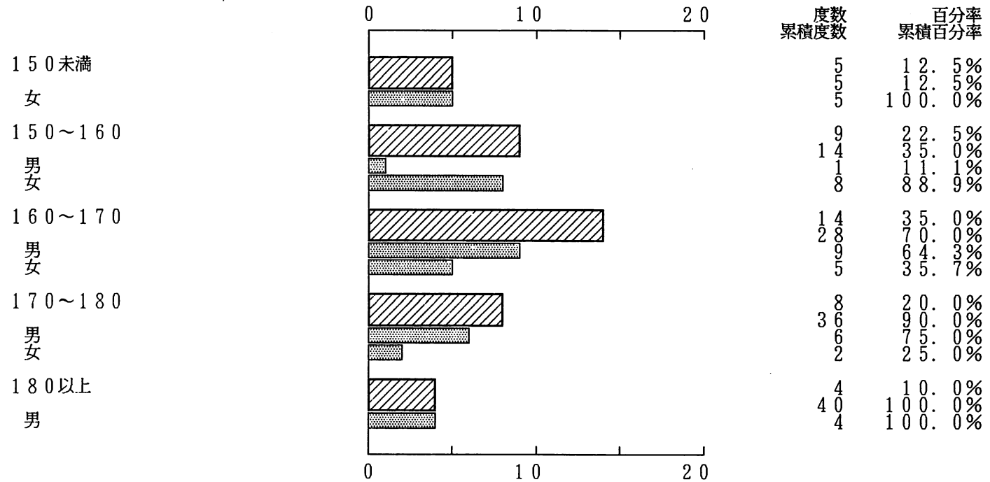
図1.20 出力結果
