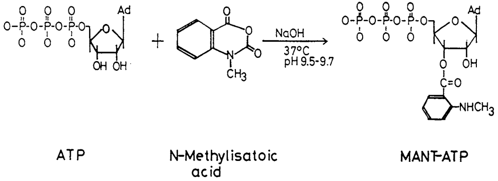
図Ⅱ-1. ATPのN-メチルアントラニル酸エステル(MANT-ATP)の合成法
