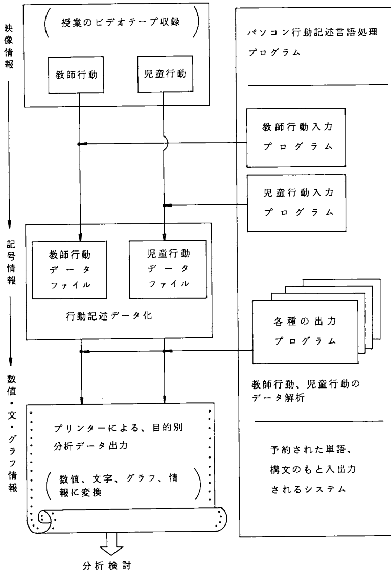
図3 個性化授業分析システムの概要
