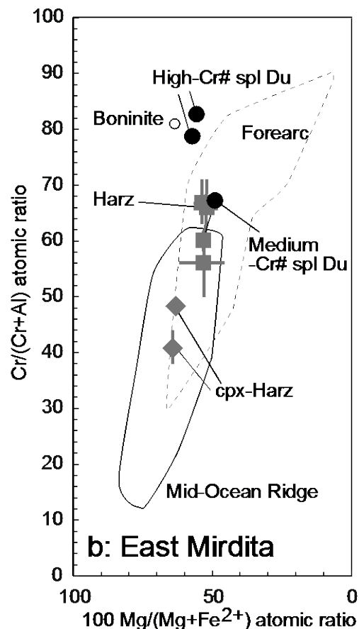
図 1. ミルディータオフィオライト東帯のかんらん岩中のスピネルの特徴
