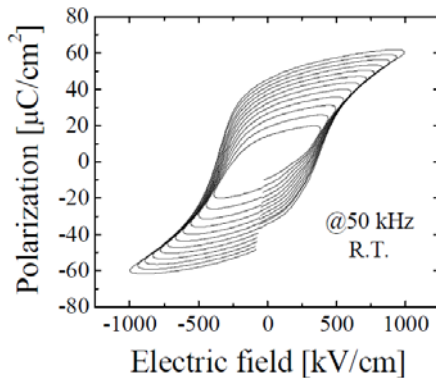
図4 試料の P-E 特性
