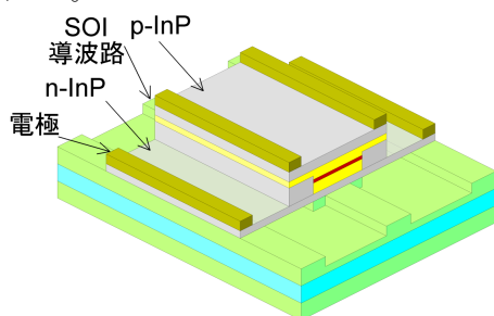
図 1 半導体薄膜レーザの電流注入構造
