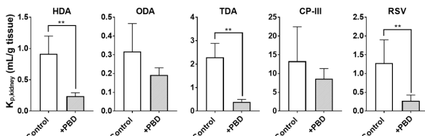
図3 胆汁カニューレ非処置ラットにおけるOATP1Bs内因性基質及びRSVの腎臓-血液間分配係数 ( K_{p,kidney} ) へのPBDの影響
