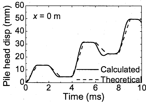
図4 変位の時間的変化
