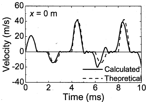
図3 速度の時間的変化
