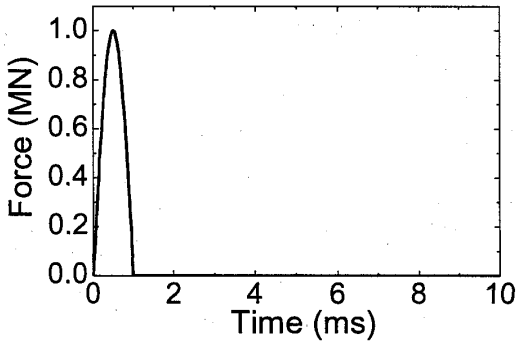
図2 杭頭載荷荷重
