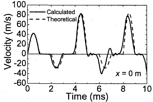
図5 速度の時間的変化
