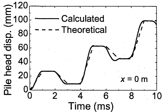
図6 変位の時間的変化
