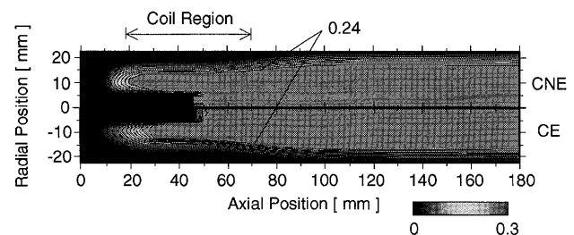
Fig. 2 大気圧 \text{Ar-O}_2 誘導熱プラズマにおけるO原子の質量分率[10].
