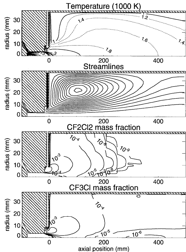
Fig. 1 PLASCONにおける温度、流線および \text{CF}_2\text{Cl}_2 、 \text{CF}_3\text{Cl} の質量分率[7].
