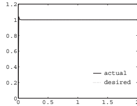
(d) Trajectory of \tilde{f}_2
