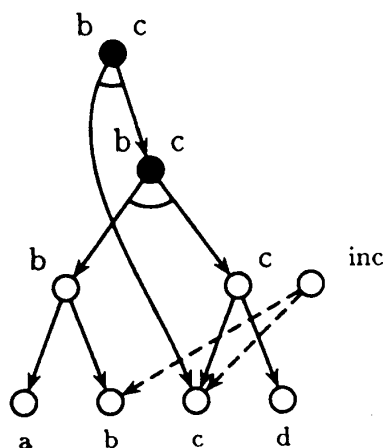
図 4: アルゴリズムの実行例
