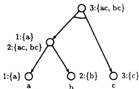
図3: ステージを用いた仮説合成の例
