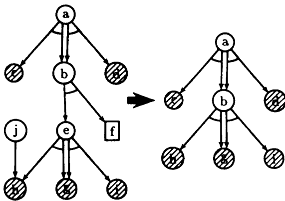
図 2: 推論パスの生成例
