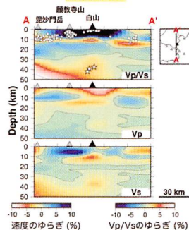
白山周辺の3次元地震波速度構造
