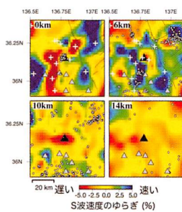
白山周辺の3次元地震波速度構造
