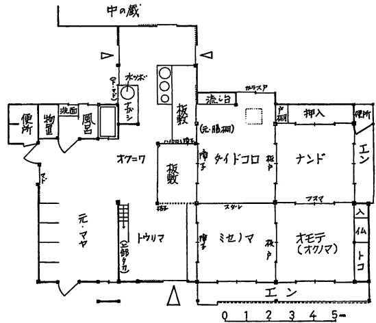
図4 (C農家) Cさん宅(久美浜町)現状図一明治28年新築一
