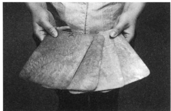
図11. 線量調節用金属板 材質：アルミニウム 大きさ：12.5×17.7cm 厚さ：0.5mm 3枚 1mm 2枚 2mm 2枚
