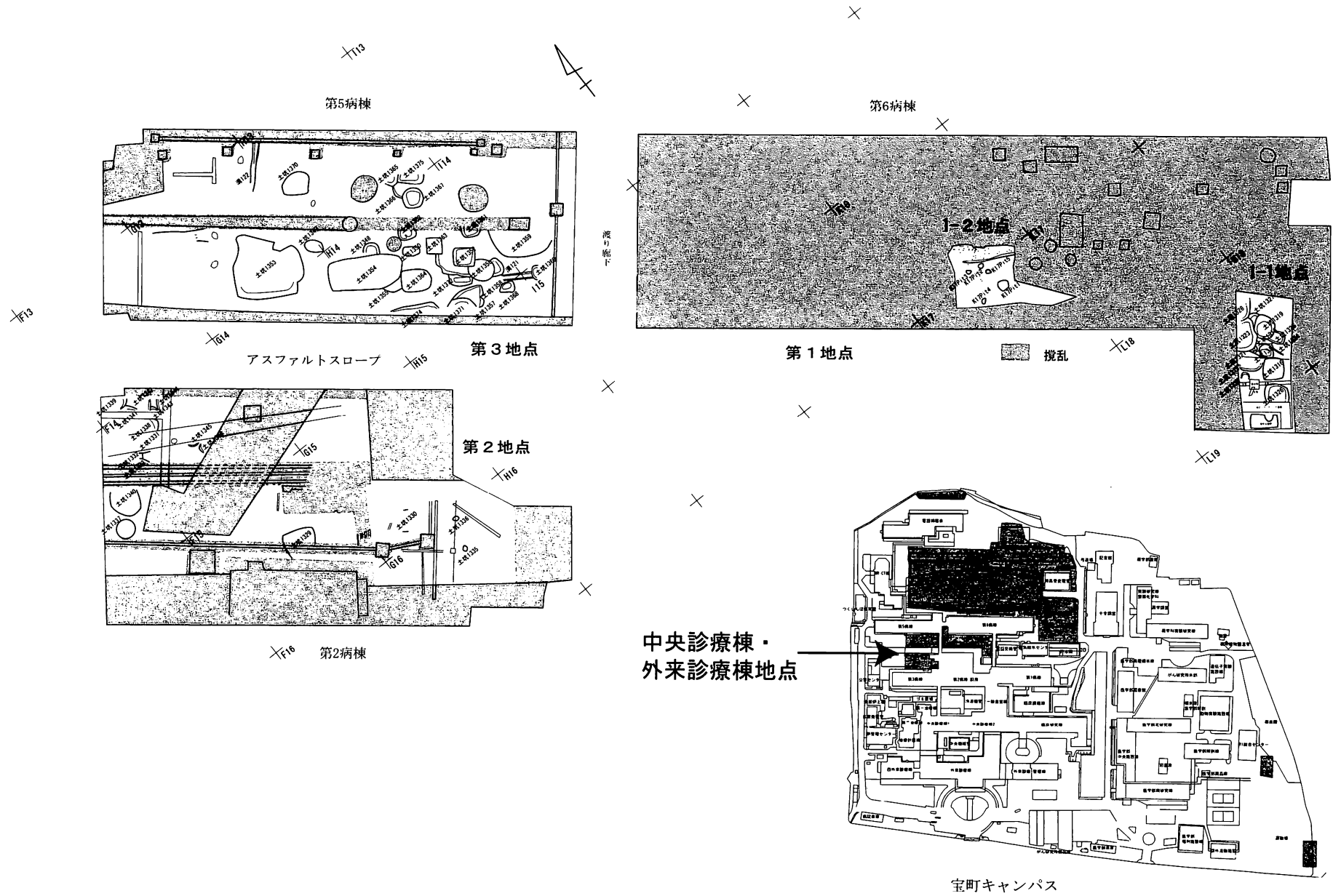
第6図 中央診療棟地点平面図(1/400)
