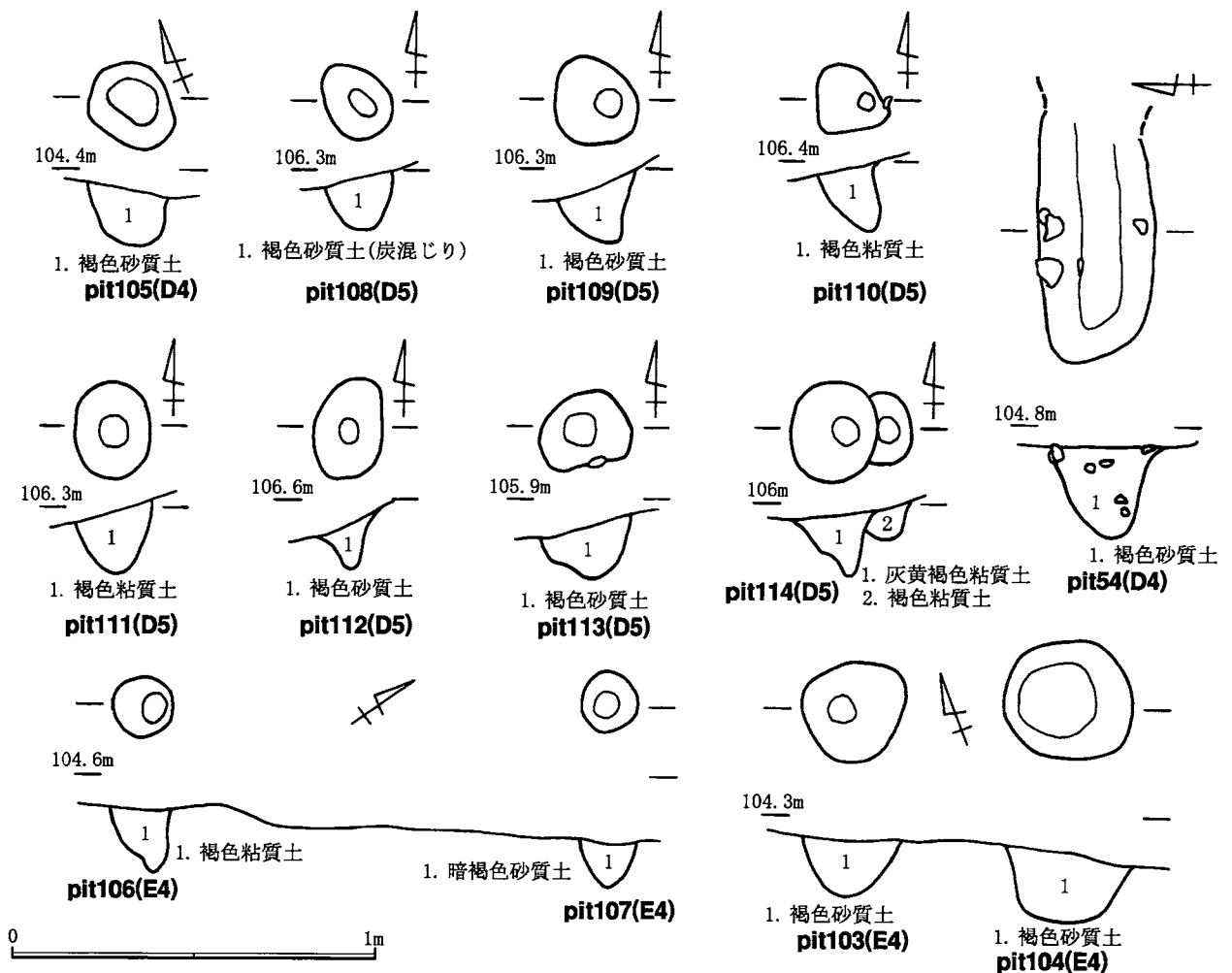
第14图 D4, D5, E4区遺構平面・断面图
