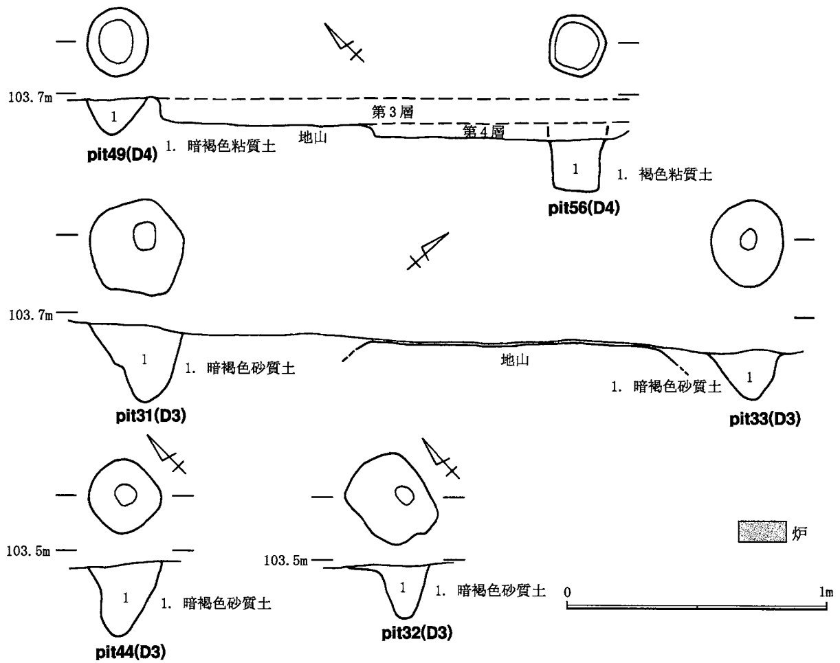
第12图 建物1pit平面・断面图
