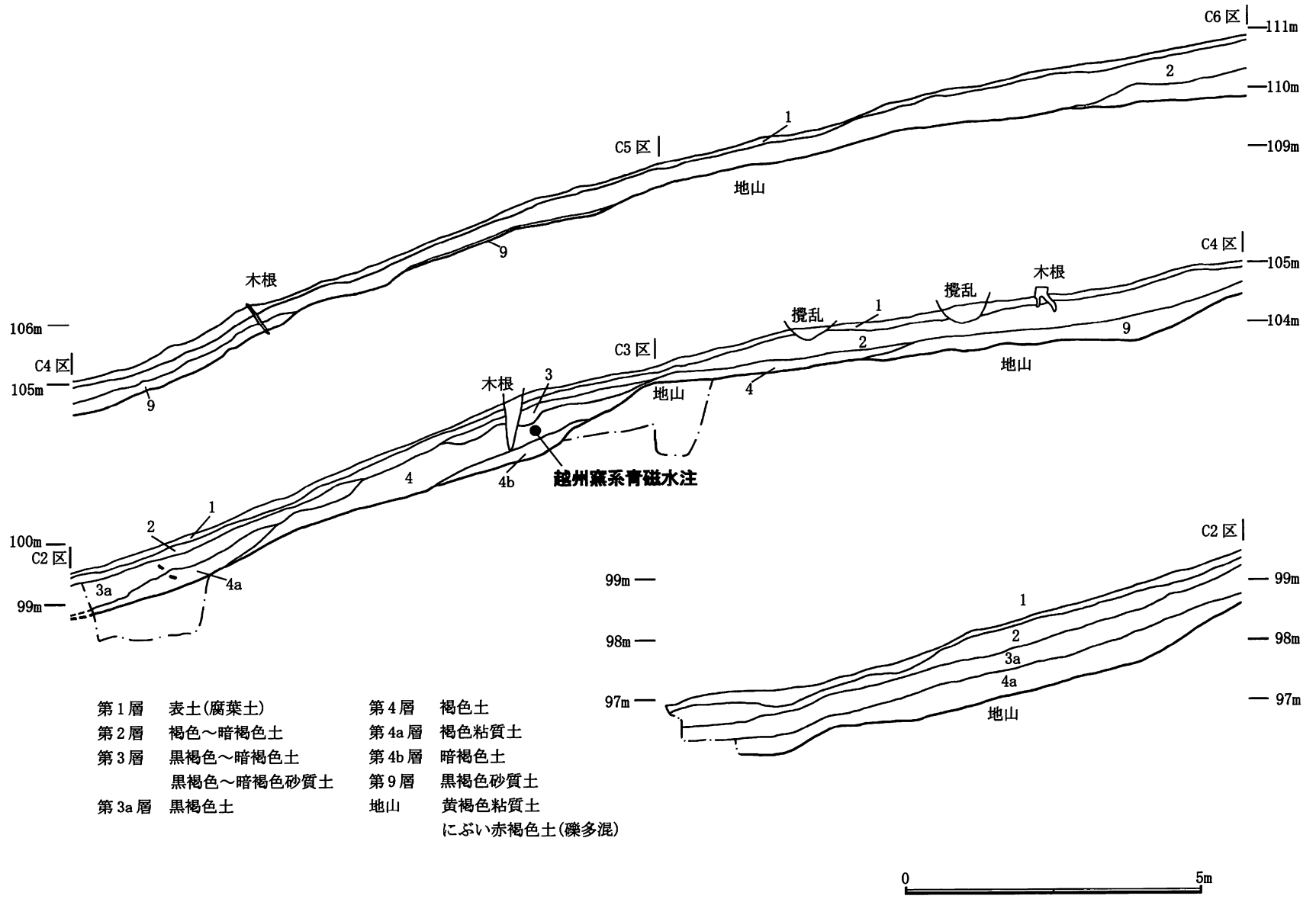
第24図 Cラインセクション図
