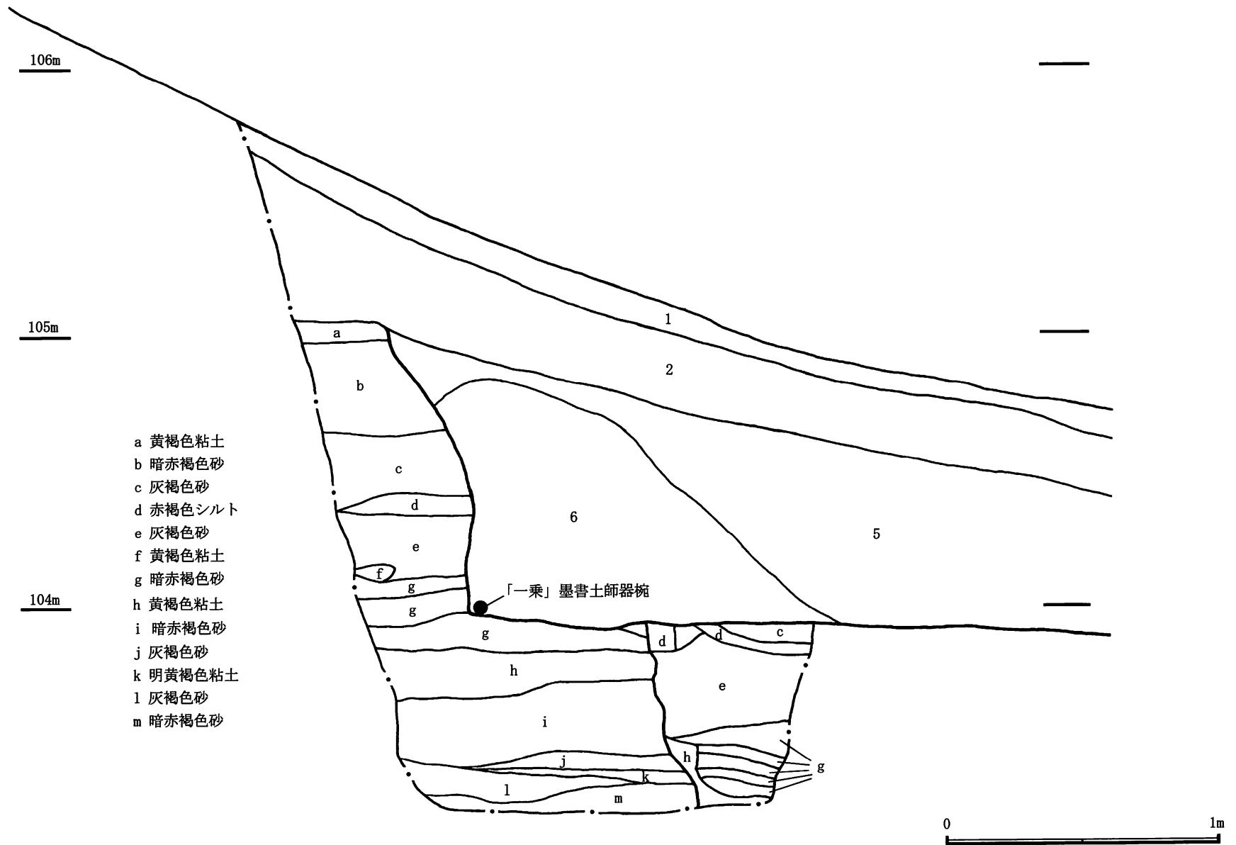
第27図 3ラインセクション図地滑り・山際削平部分(F3区)
