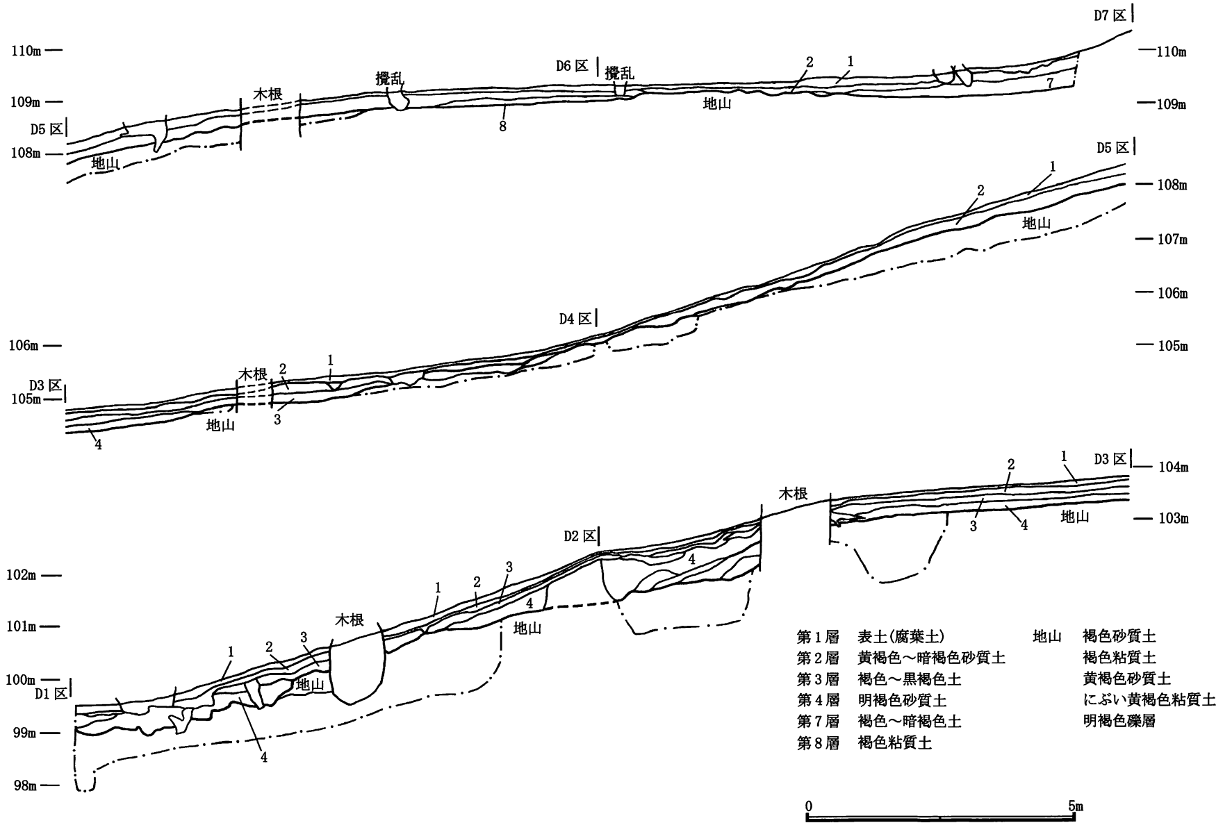
第23図 Dラインセクション図
