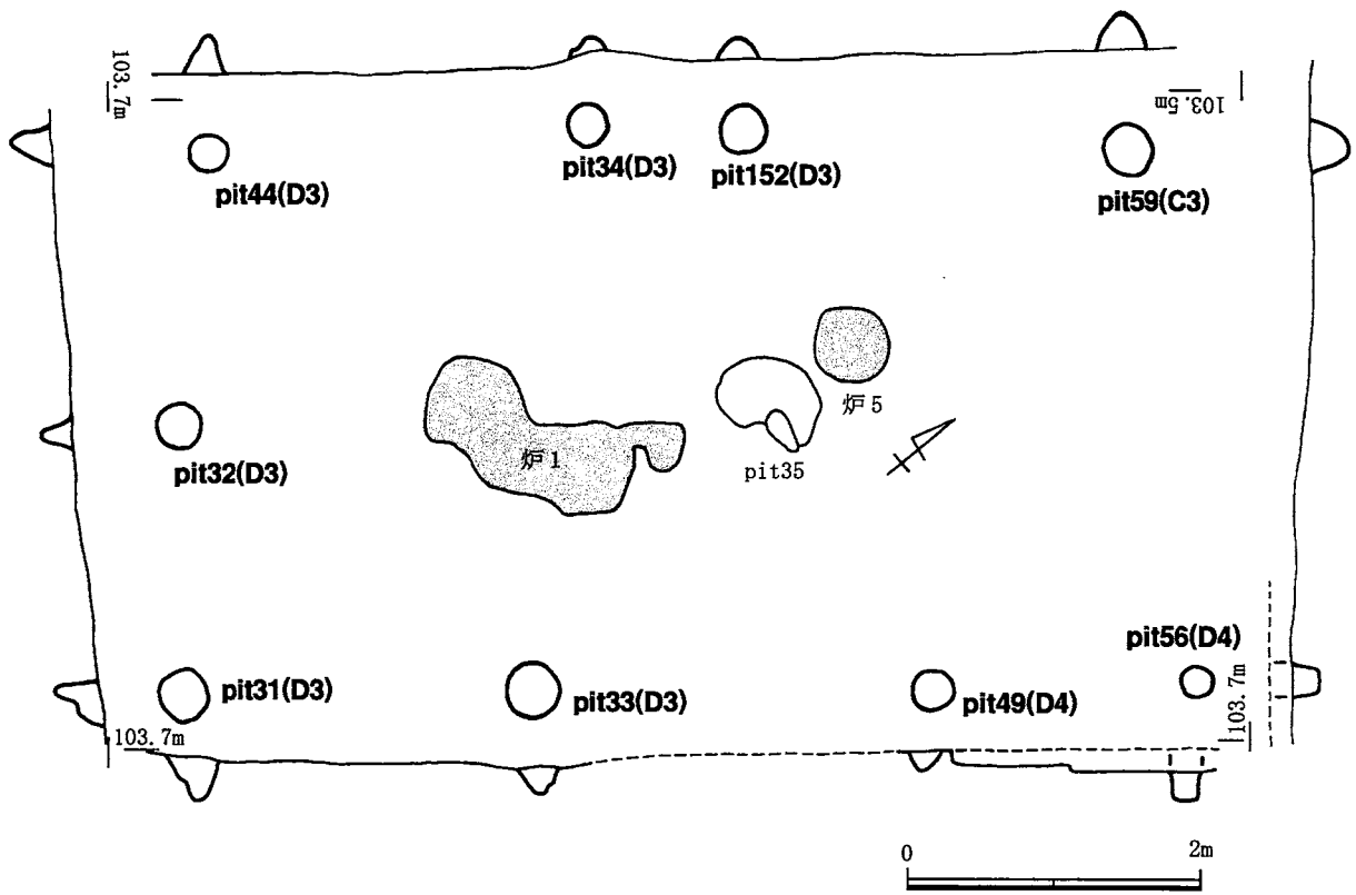
第11图 建物1平面・断面图
