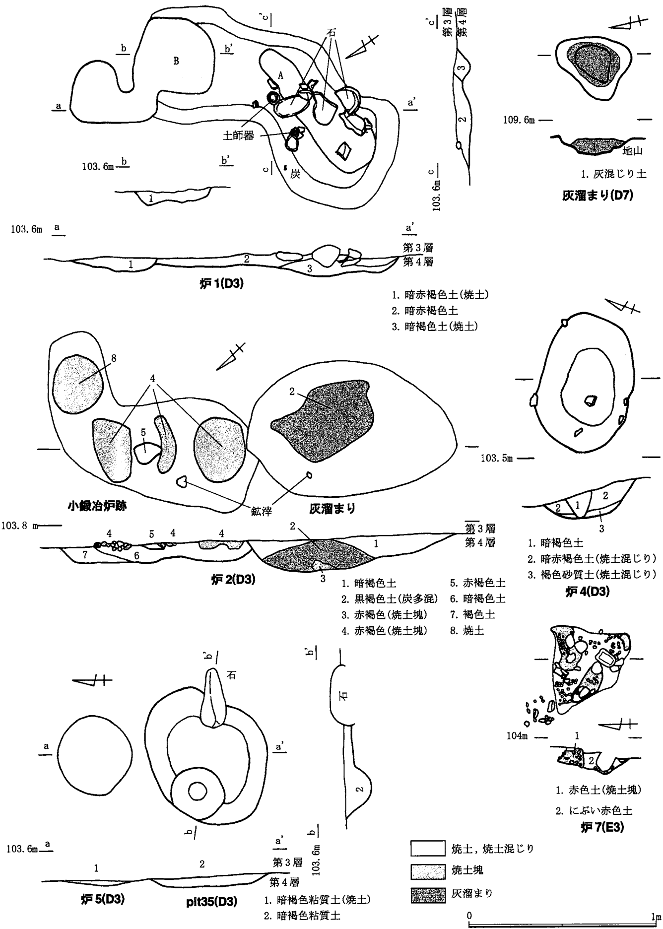
第10図 炉1, 2, 4, 5, 7, pit35, 灰溜まり平面, 断面図
