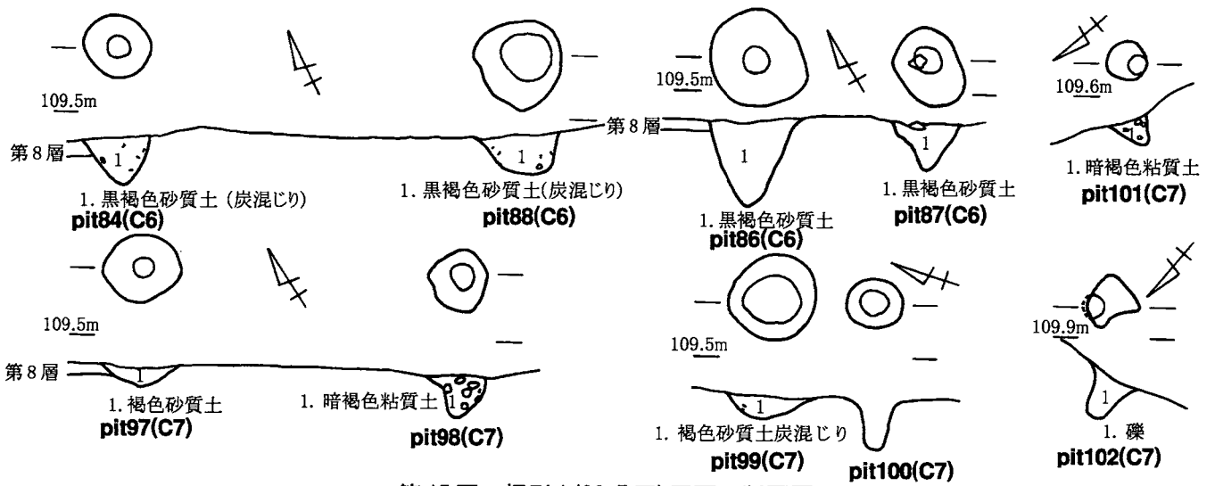
第15図 柵列1 (C6, 7区) 平面・断面図
