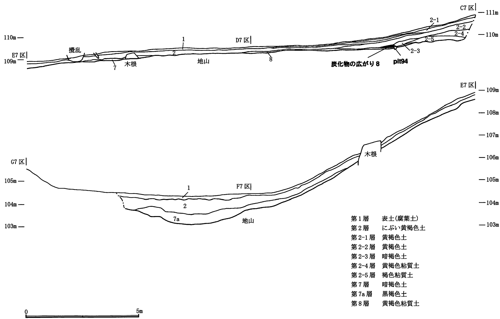
第28図 7ラインセクション図
