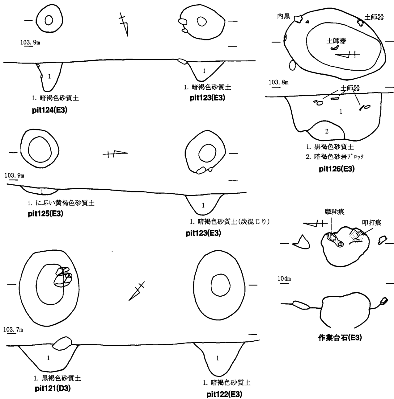
第17図 D3, E3区遺構平面・断面図
