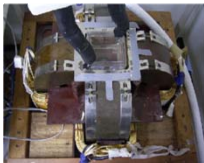
図1 60Hz 交流磁界発生装置
