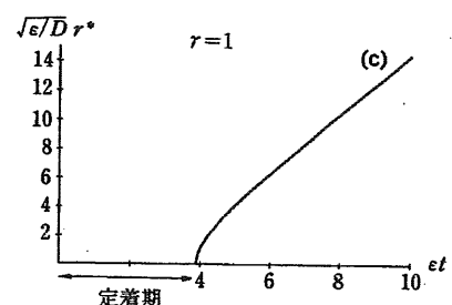
図3.4 Skellamモデル(3.10)から導かれる伝播距離-時間曲線(3.14)式を \gamma = \varepsilon N_0 / Dn^* = 10, 2.5, 1 の場合についてプロットした。縦軸は R = \sqrt{\varepsilon/D} r^* 、横軸は T = \varepsilon t を表わしている。 \gamma < 4.6 のときにのみ定着期が現われる。 \gamma の減少に伴って定着期は長くなるが、いずれの場合もタイプ1の伝播パターンを示す。
