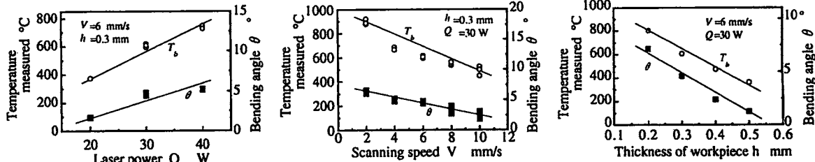
図7 レーザフォーミング加工における加工条件の影響
