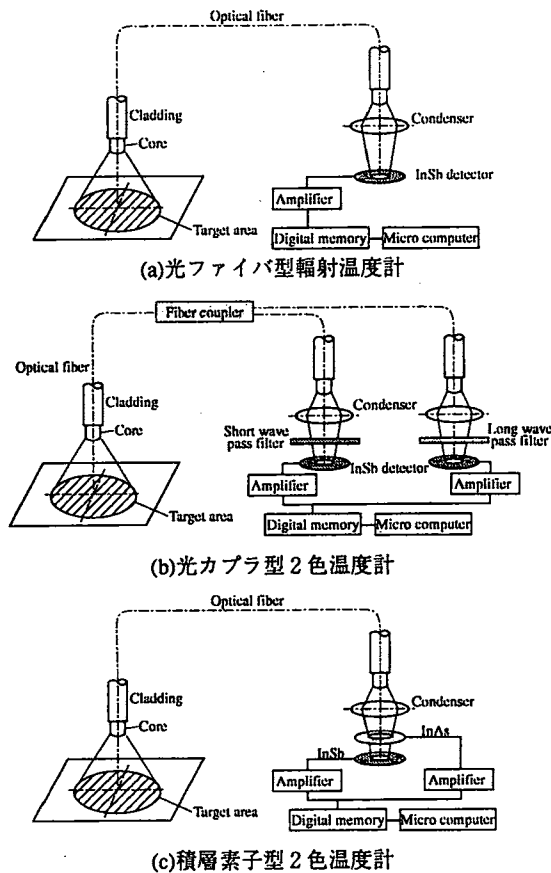
図1 温度計概略
