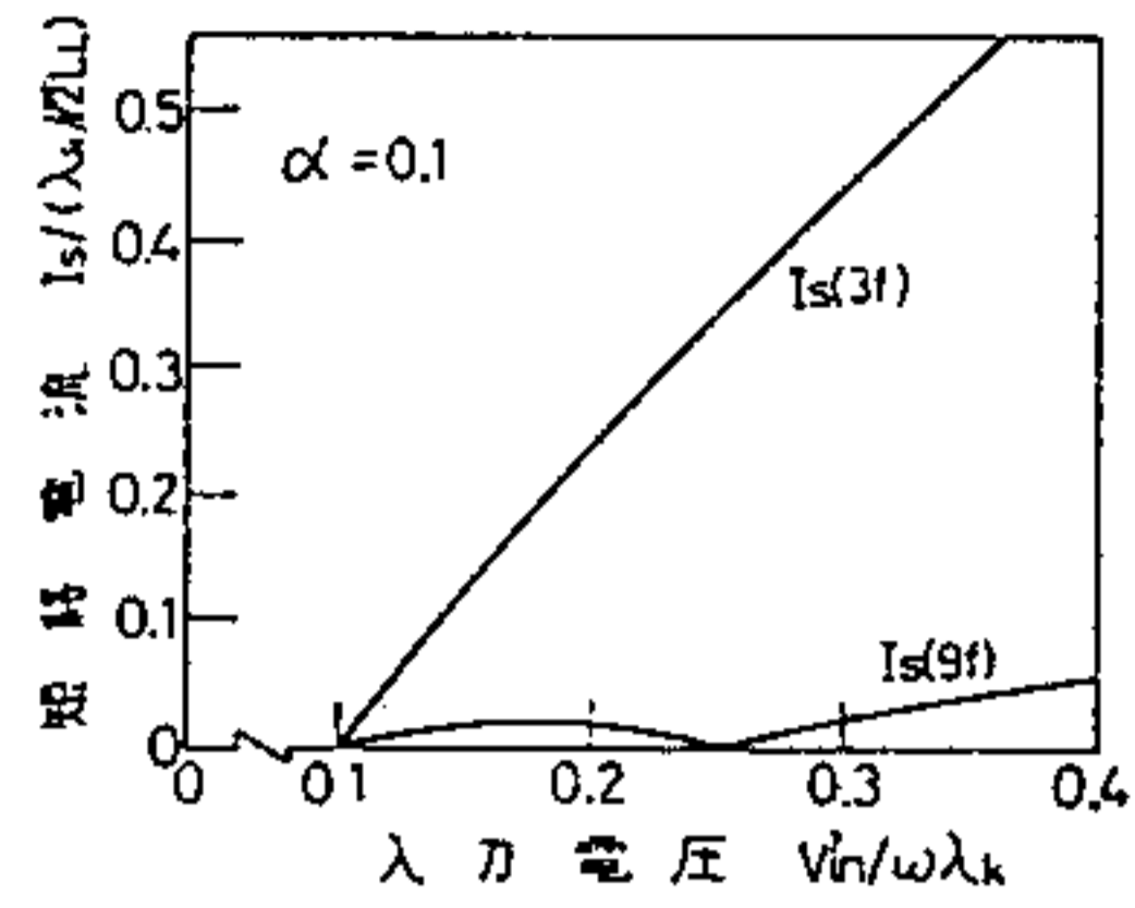
(a) 二次側短絡電流
