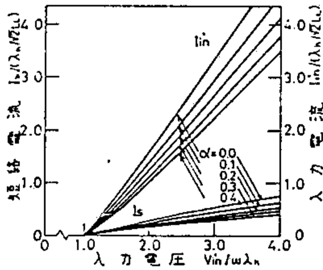
第 11 図 短絡時の特性
