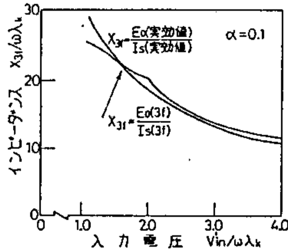
第 13 図 二次側の等価リアクタンス X_{3f}
