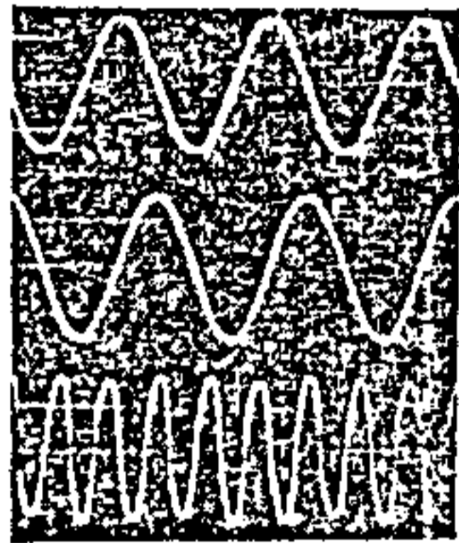
Vin=160V, 負荷電流 2.5A
