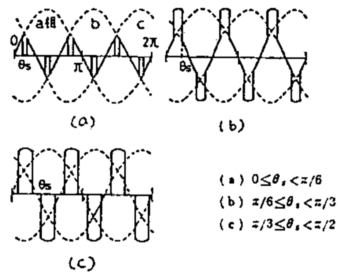
第7図 周波数変換部の出力電圧波形
