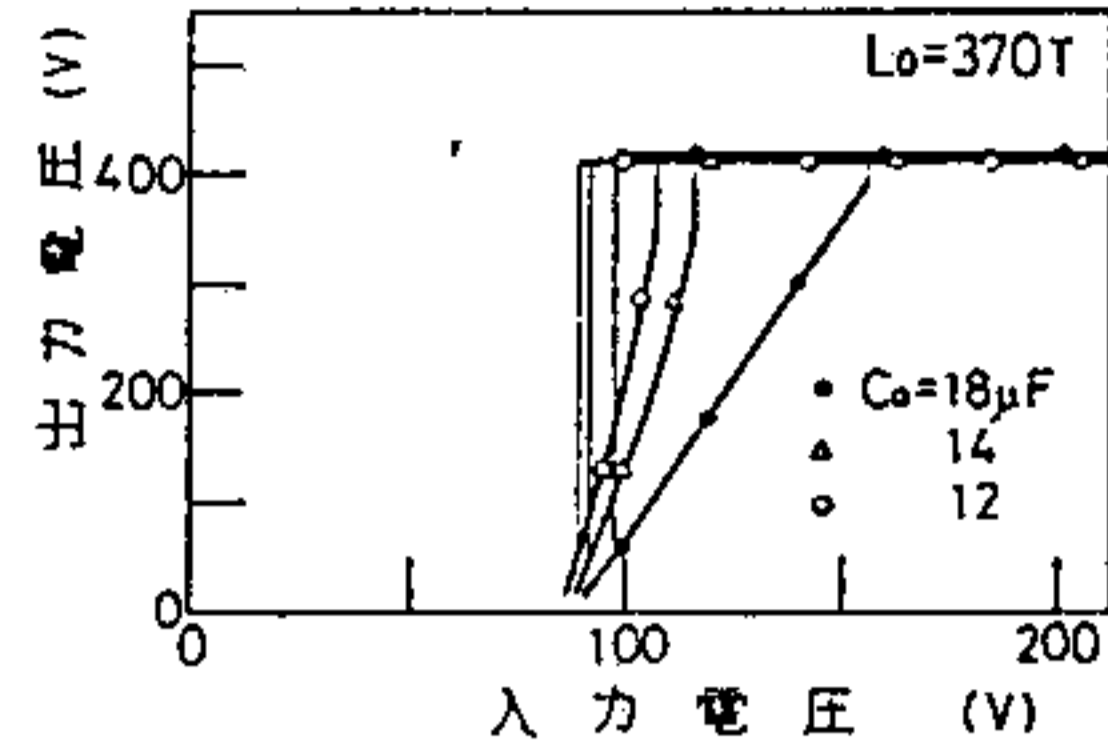
(a) C_o に対する電圧特性
