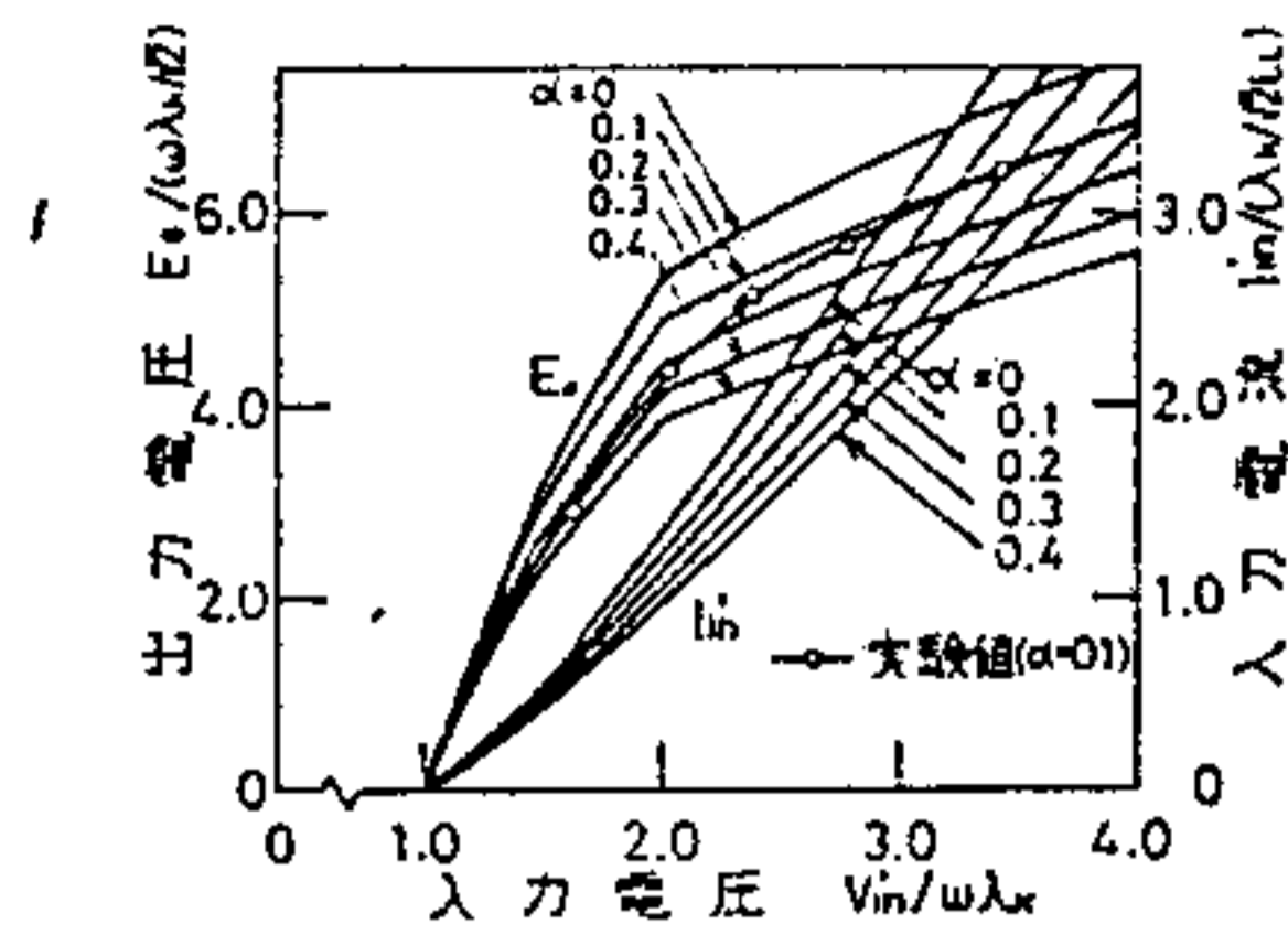
第 8 図 二次側開放時の特性
