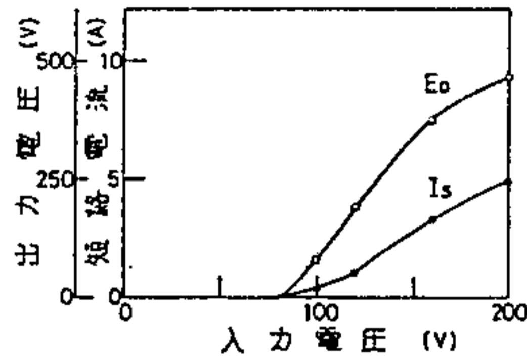
(a) 周波数変換部の出力電圧、短絡電流特性
