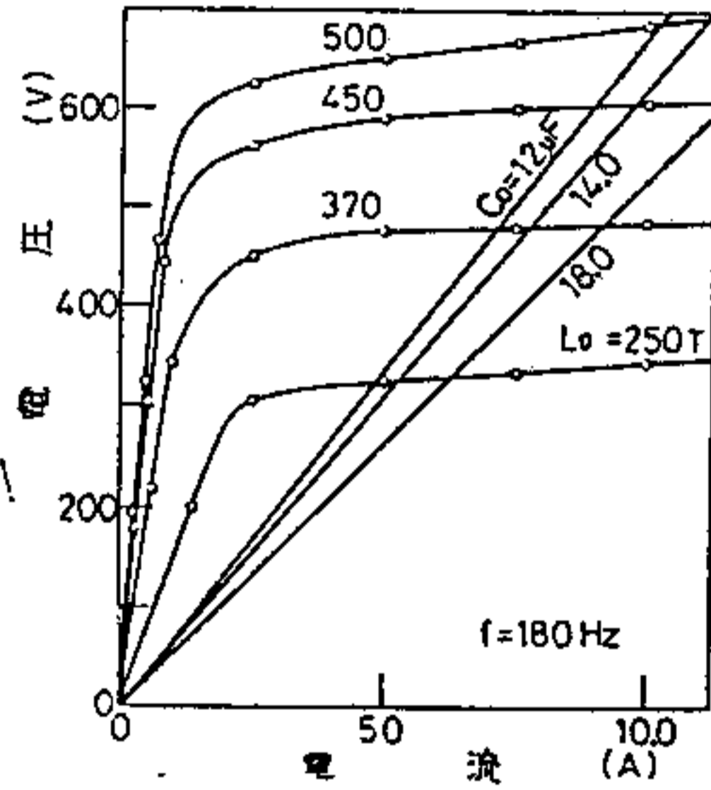
(b) 共振回路の特性
