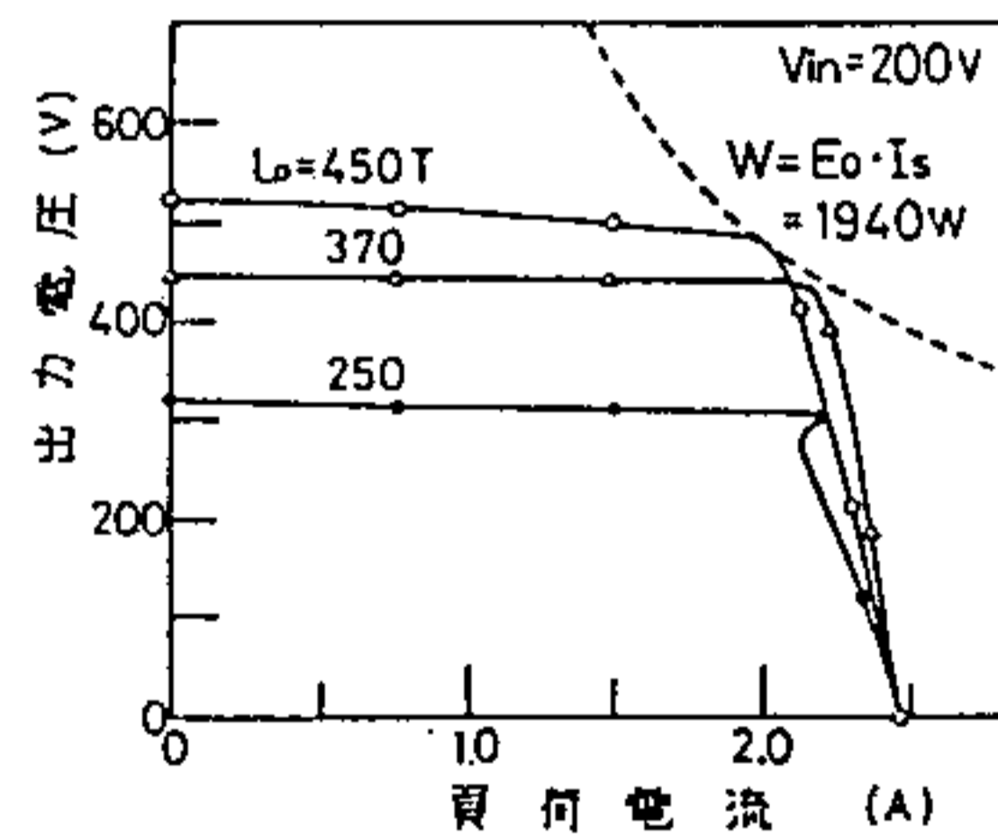
(d) L_o に対する負荷特性
