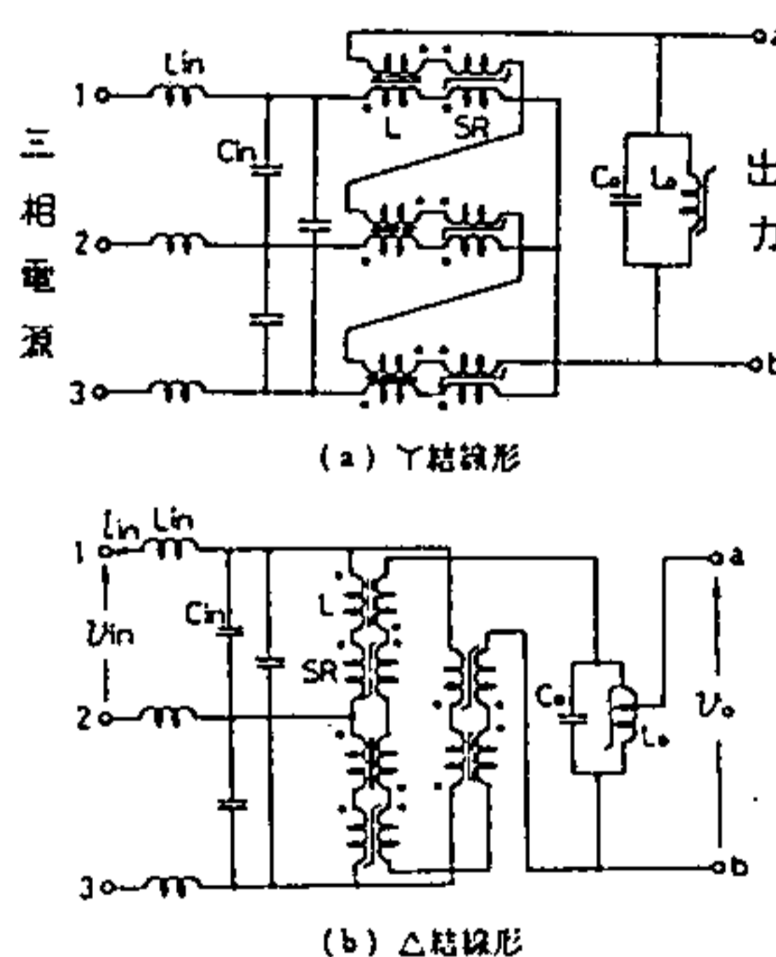
第 1 図 直列接続リアクトル回路による 3 倍周波数通倍器
