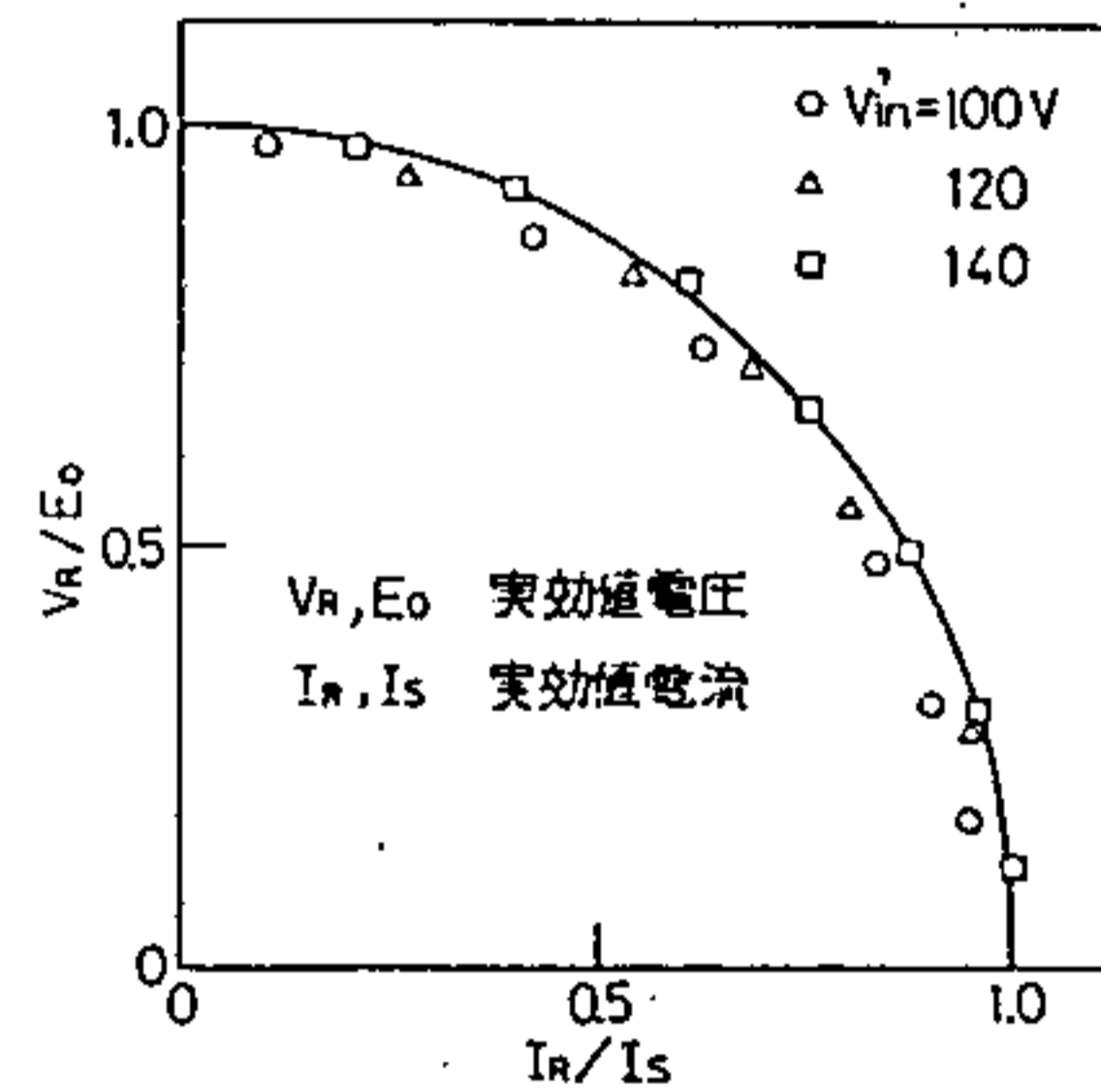
第3図 周波数変換部の負荷特性
