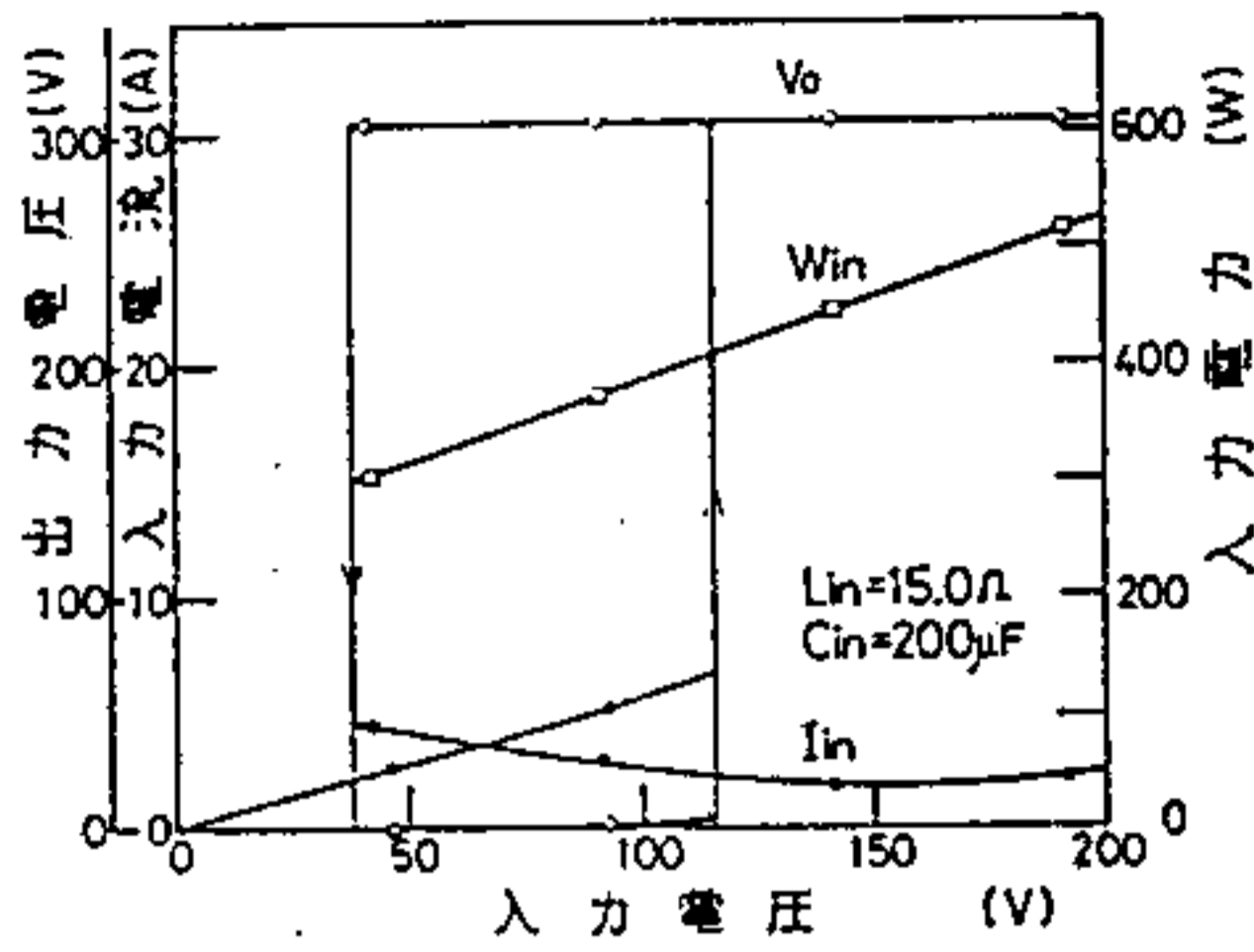
(a) 電圧特性
