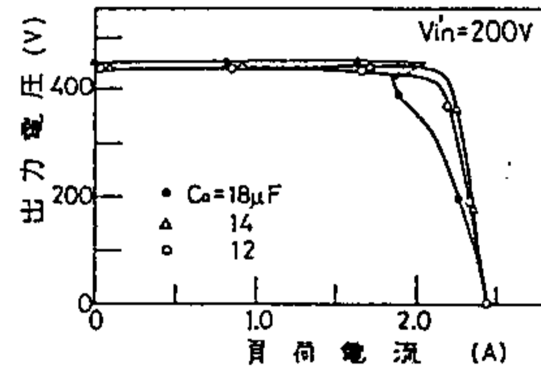
(b) C_o に対する負荷特性
