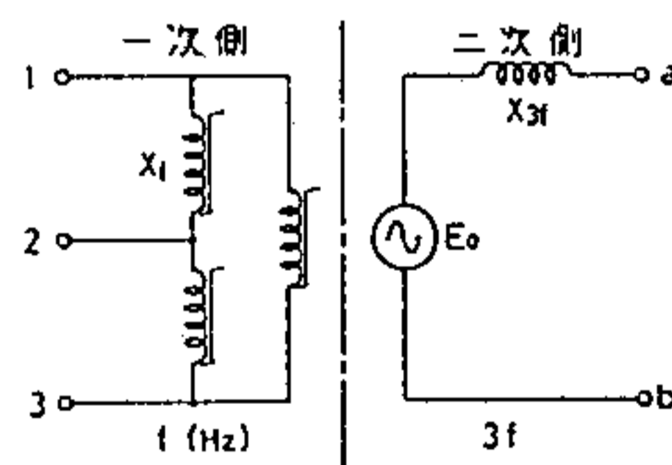
第4図 周波数変換部の等価回路
