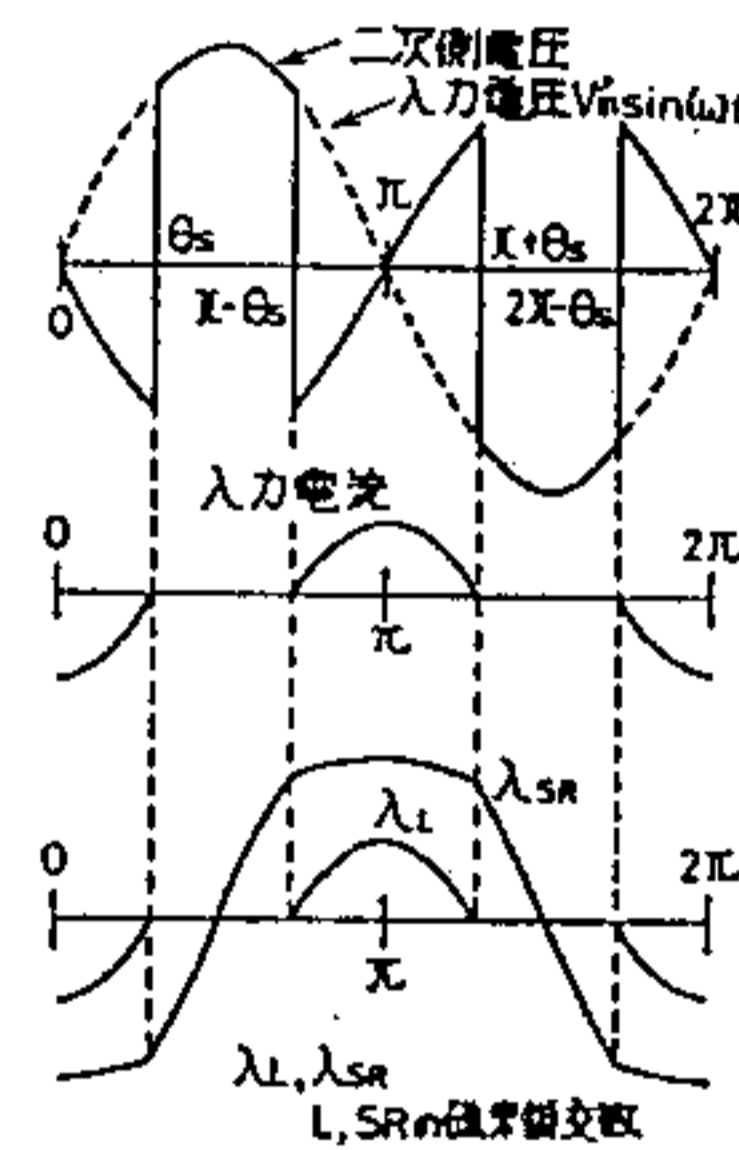
第6図 直列接続リアクトル回路の各波形
