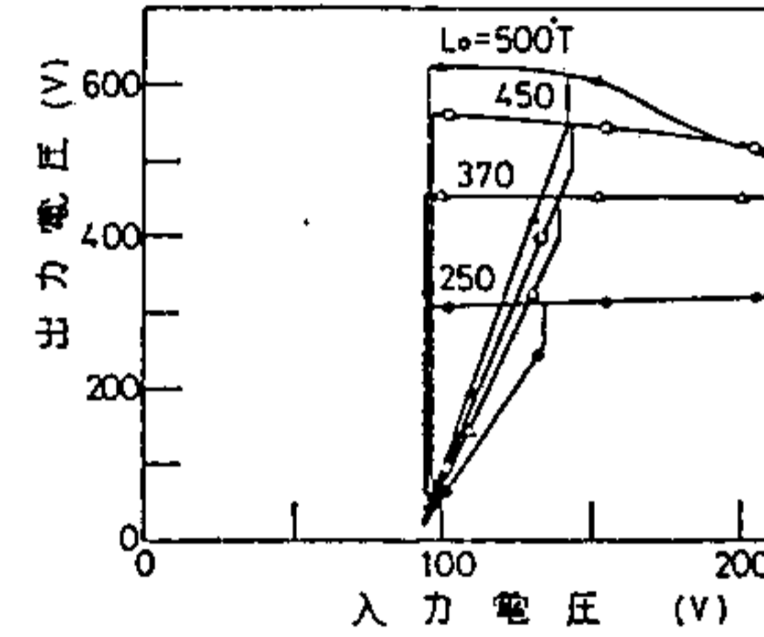
(c) L_o に対する電圧特性
