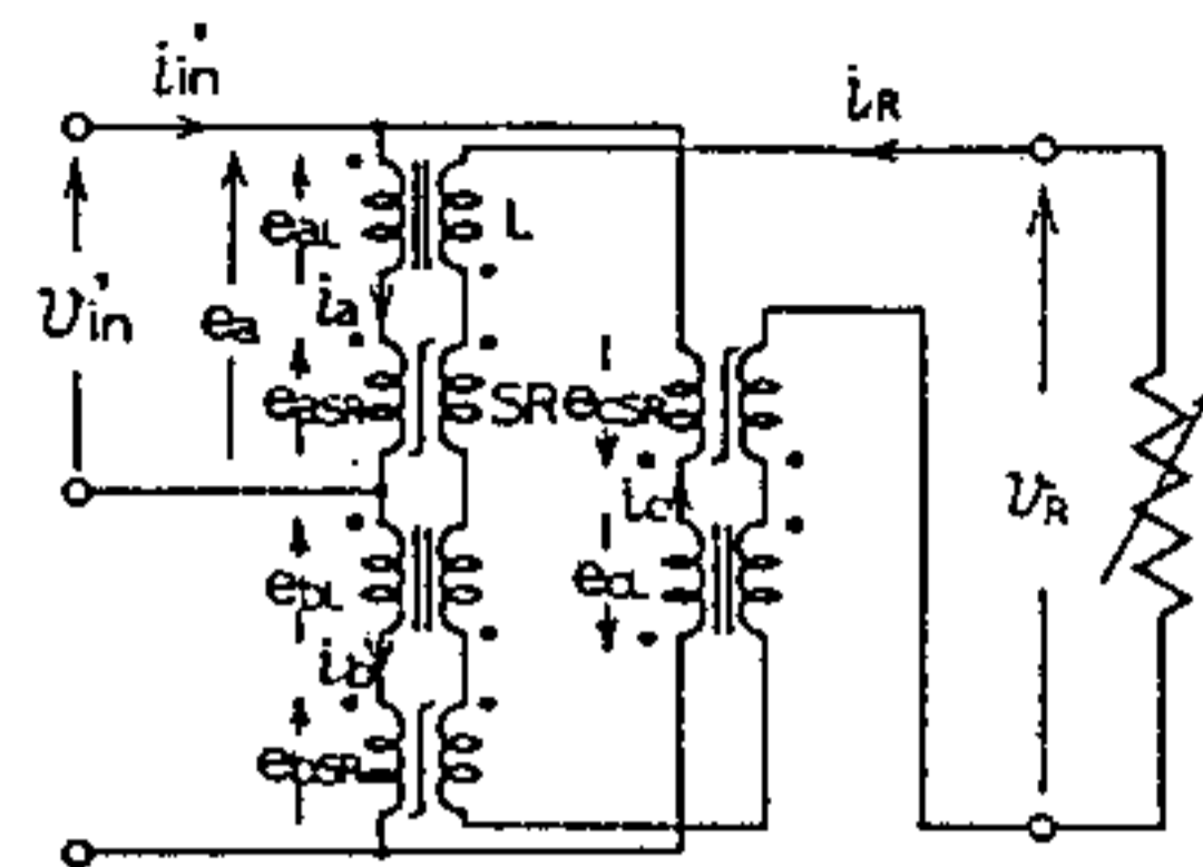
L, SR の巻数比(一次/二次側) = 1
