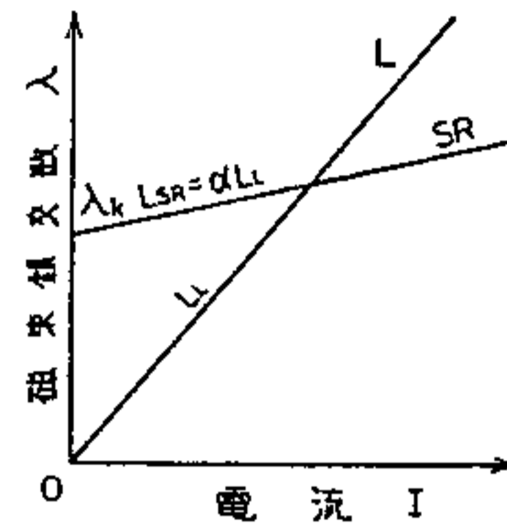
第5図 L, SR の近似
