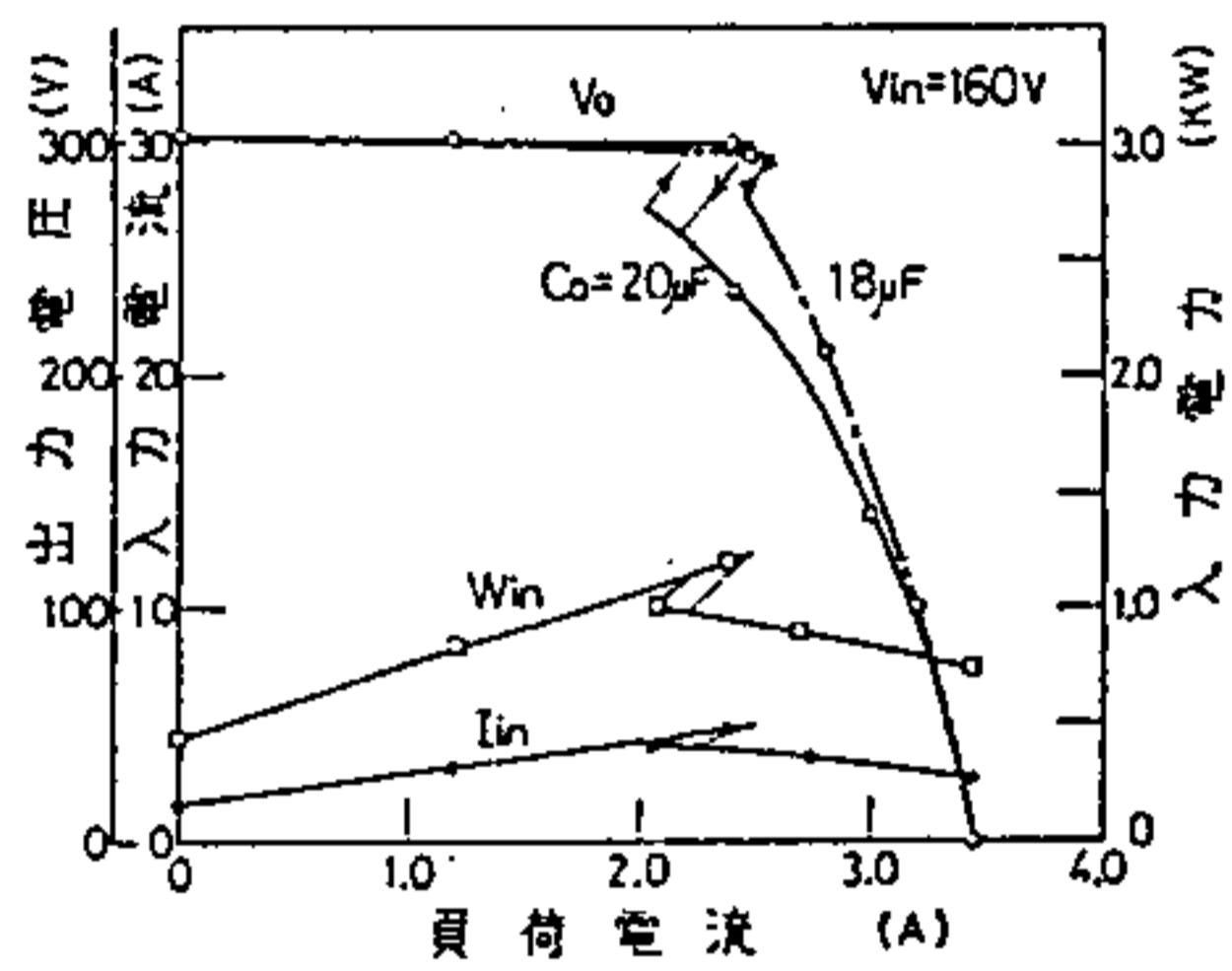
(b) 負荷特性
