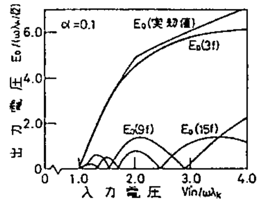
(a) 二次側開放電圧
