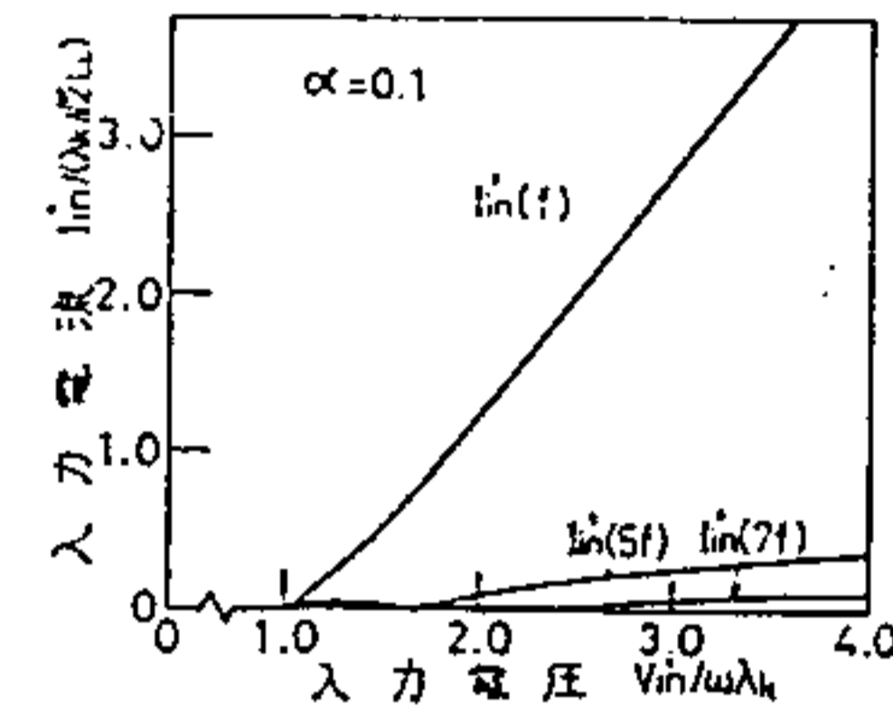
(b) 一次側入力電流
