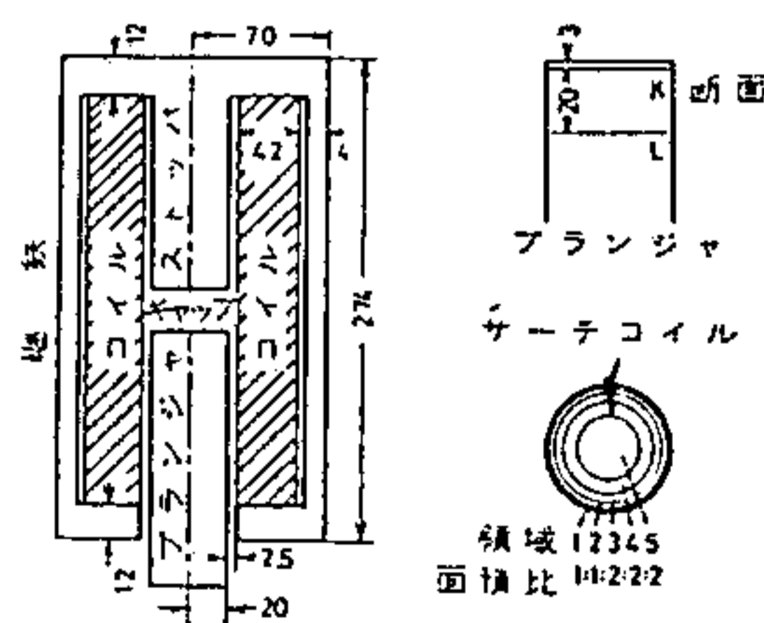
第1図 プランジャ形直流電磁石
