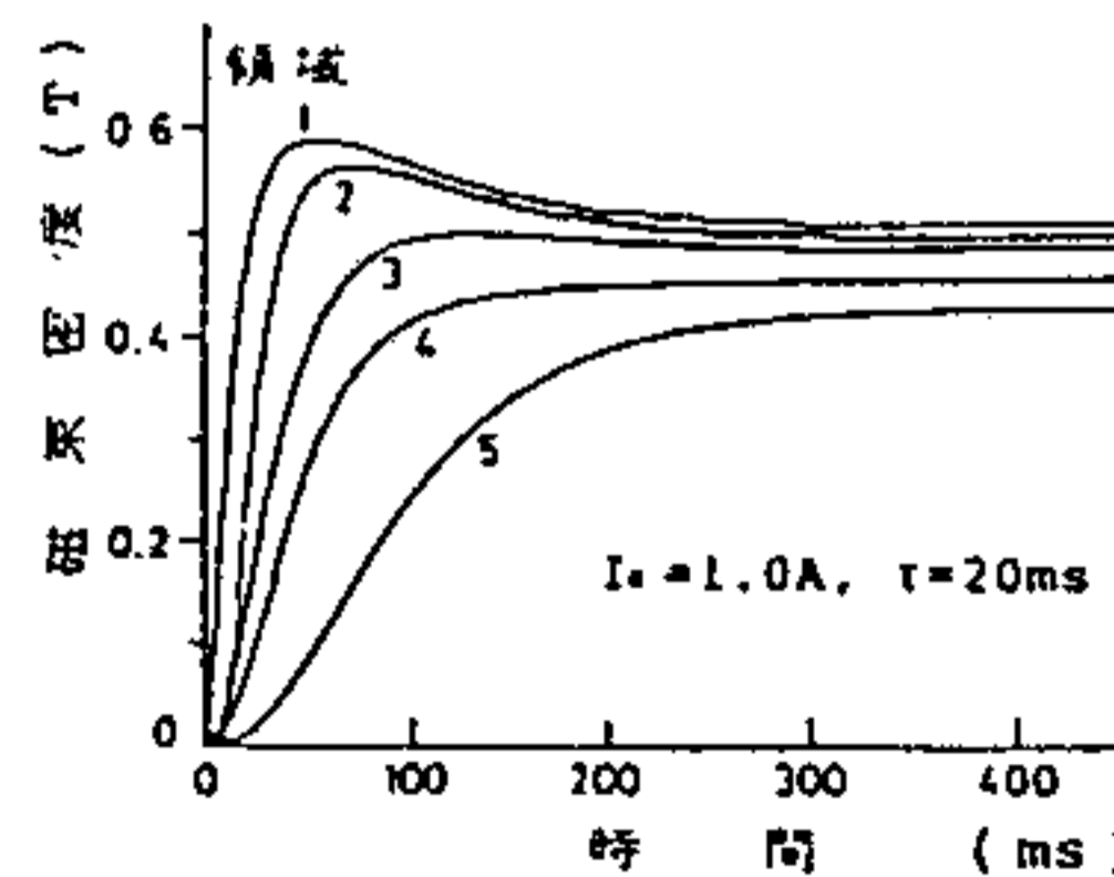
第8図 L断面の磁束密度の応答
