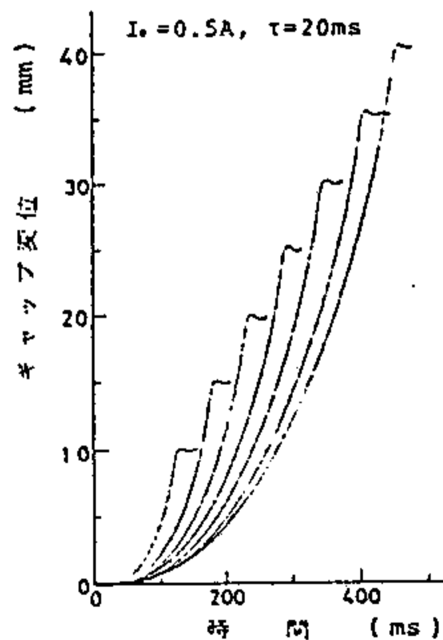
第13図 プランジャの動作曲線 Fig. 13. Operation curves of the plunger.
