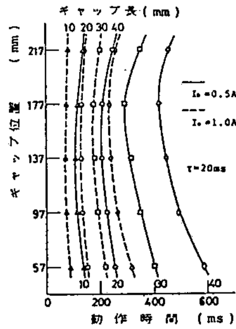
第 18 図 ギャップ位置に対する動作時間 Fig. 18. Operating time for various values of the gap position.
