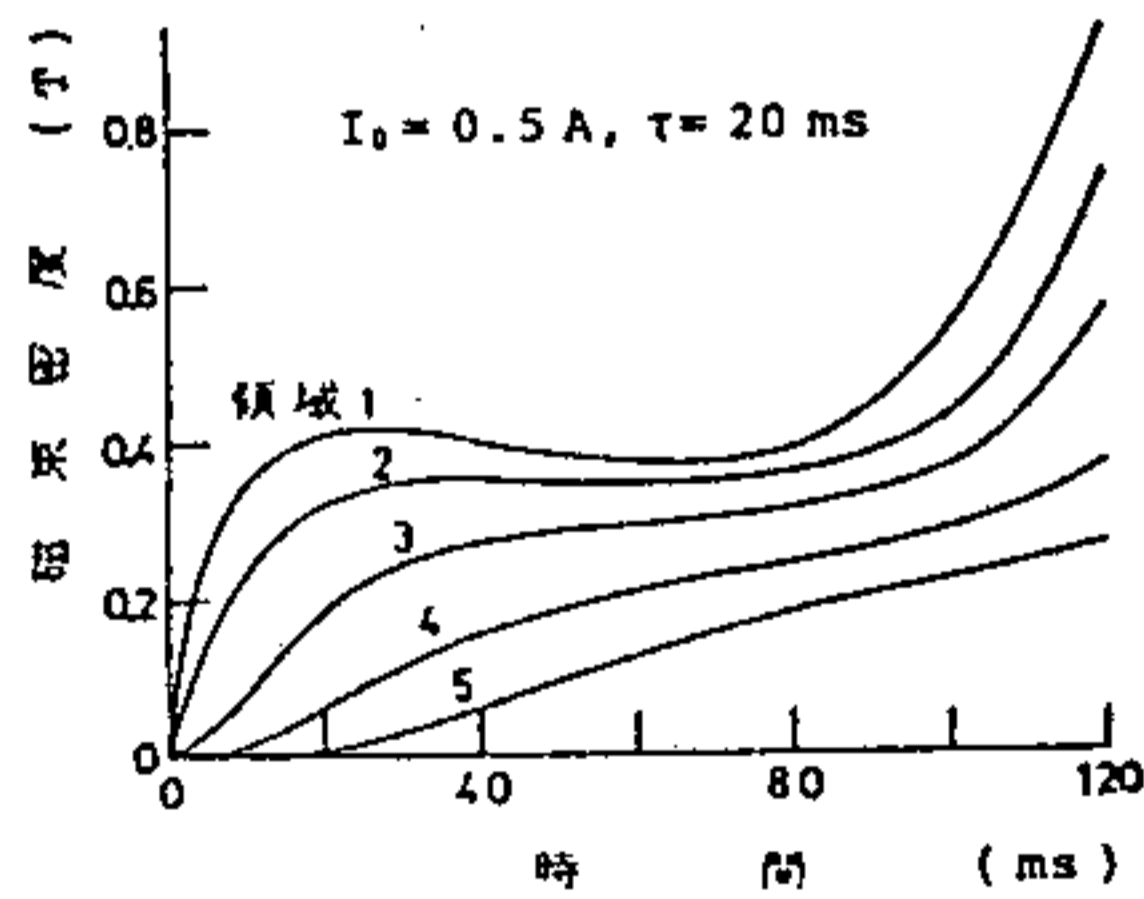
第 16 図 過渡状態の磁束密度の応答(計算値) Fig. 16. Response of the flux density at the transient state (calculated value).
