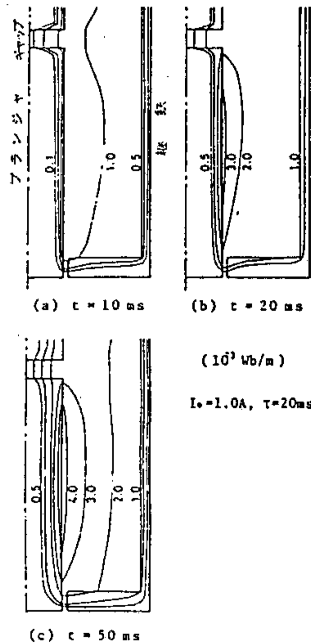
第5図 準過渡状態のベクトルポテンシャル分布
