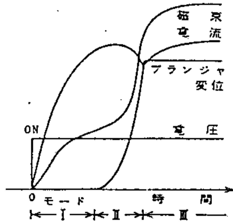
第3図 動作モード Fig. 3. Operation mode.
