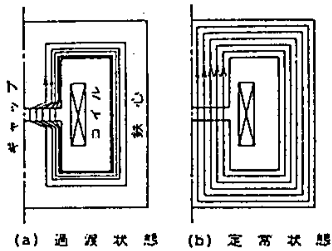
第12図 極面効果
