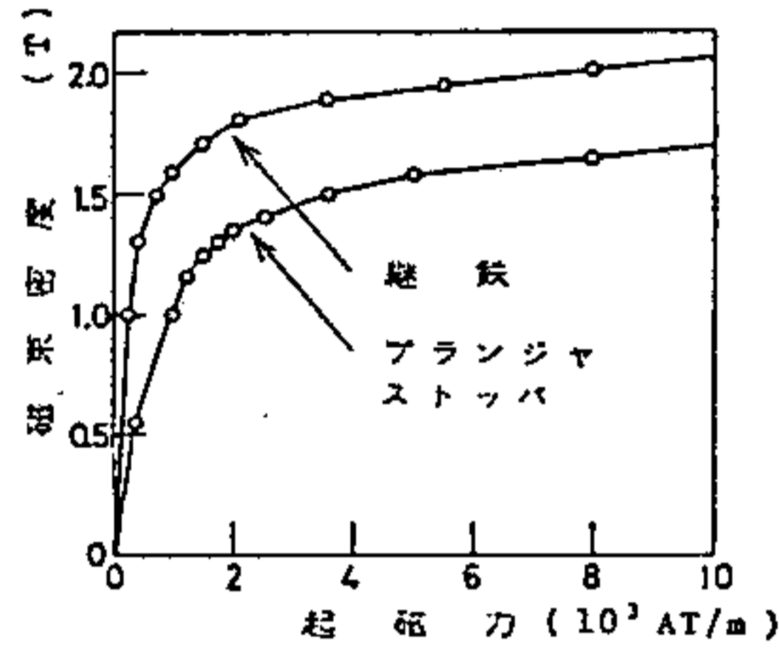
第2図 鉄心の B-H 特性 Fig. 2. B-H curve of iron core.
