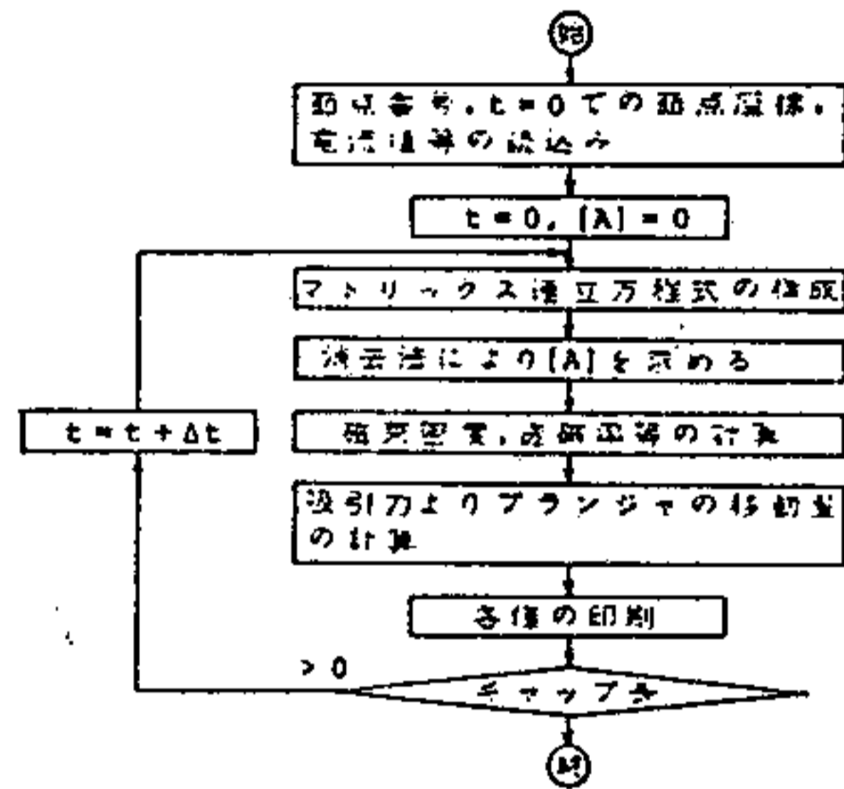
第4図 過渡状態のフローチャート Fig. 4. Flow chart for the transient state.
