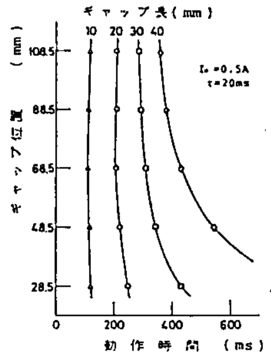
第 19 図 小形電磁石の動作時間 Fig. 19. Operating time on the small electromagnet.
