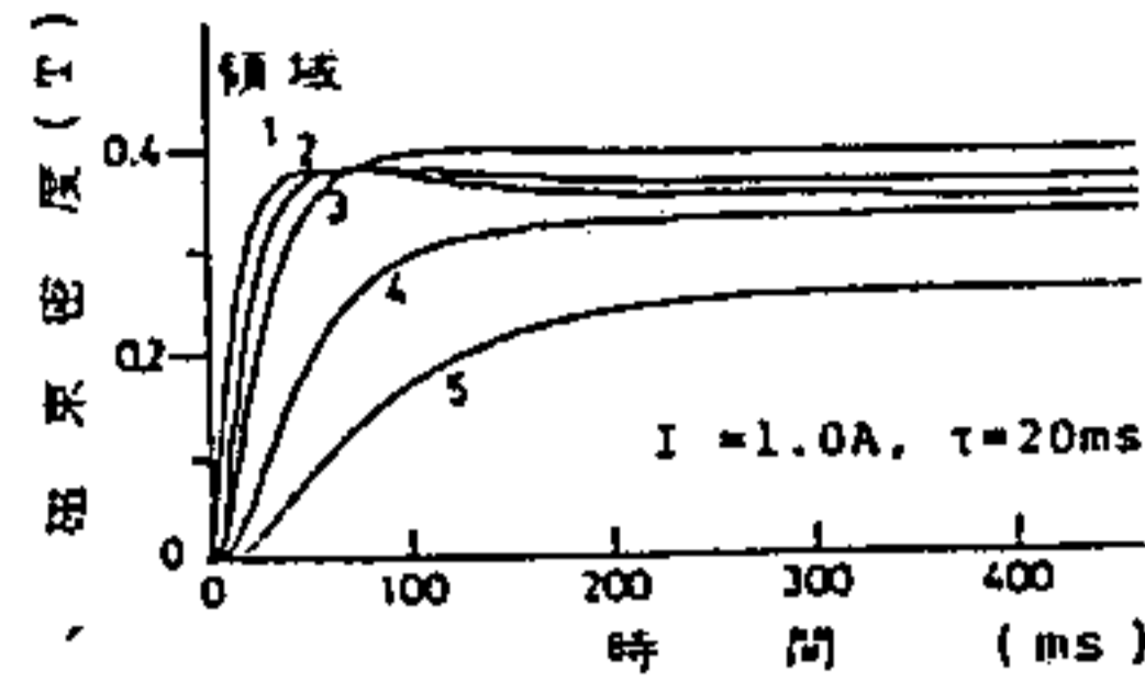
第9図 K断面の磁束密度の応答
