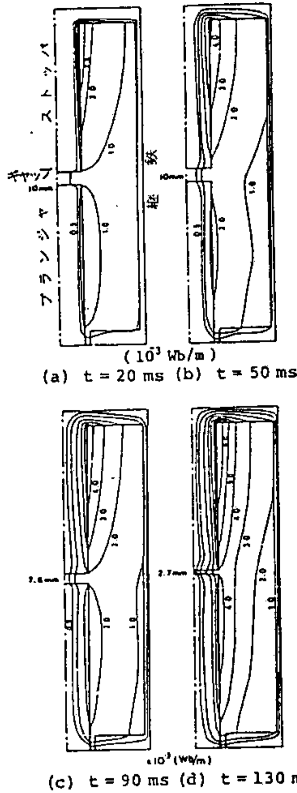
第 15 図 過渡状態のベクトルポテンシャル分布
