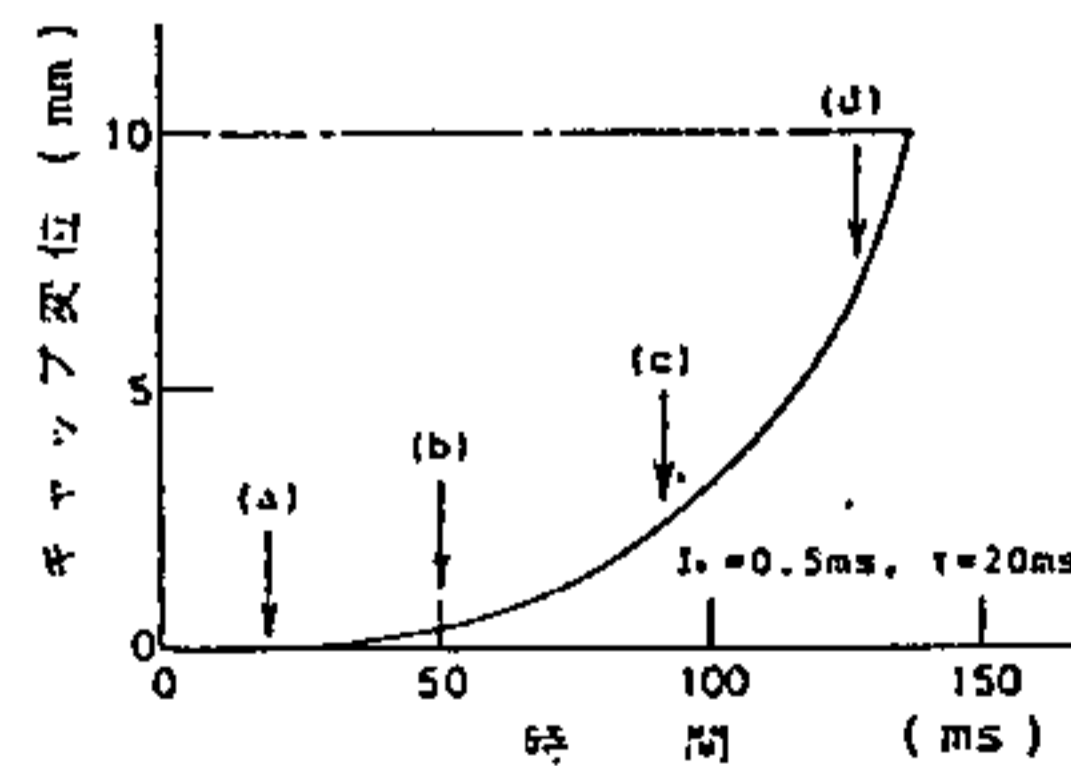
第14図 プランジャの動作曲線(計算値) Fig. 14. Operation curve of the plunger (calculated value).
