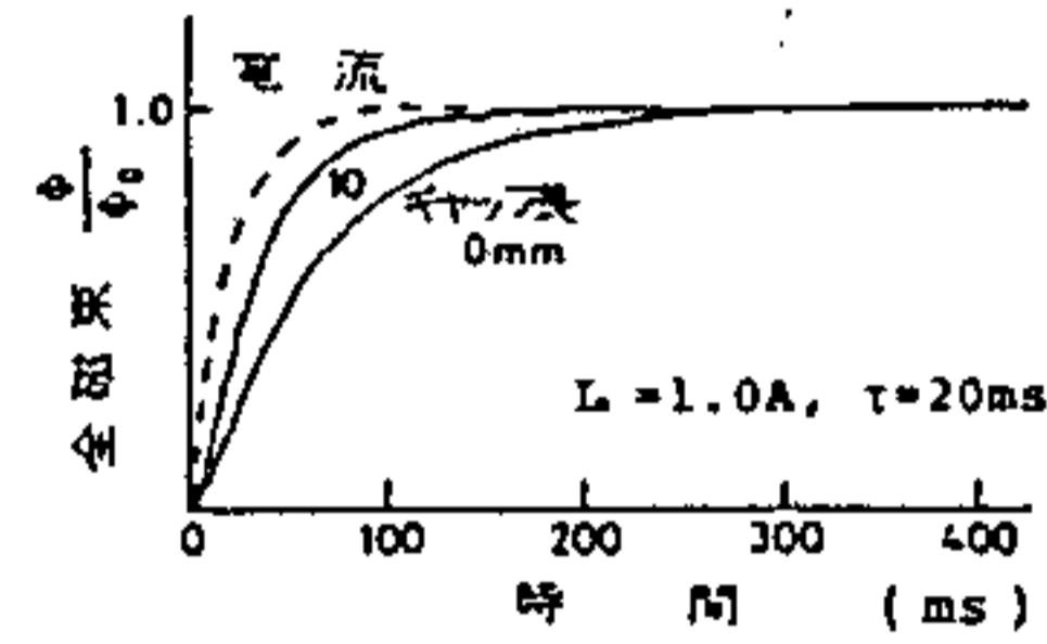
第11図 全磁束の応答
