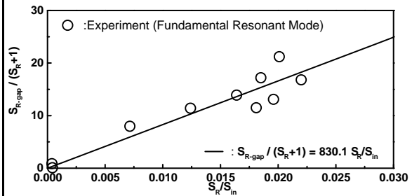
図-7 流体共振の発生規模
