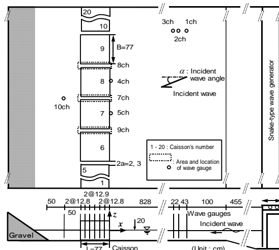
図-1 実験装置の概要（ケーソン式防波堤）
