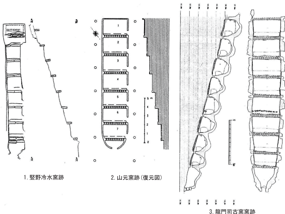
図3 薩摩焼の窯構造(2) (S=1/200)
