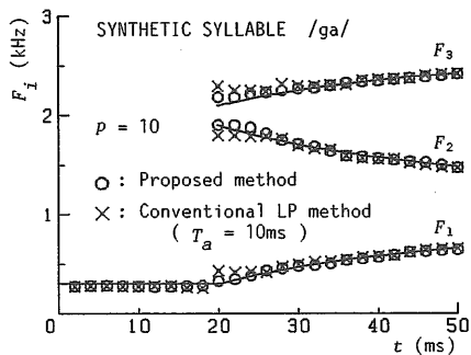
図6 ホルマント周波数軌跡推定の比較—合成有声破裂音/ga/— Fig. 6 The comparison of formant trajectory extraction for synthetic syllable /ga/.
