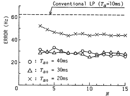
図5 ホルマント周波数推定誤差の外挿データ点数 N 依存性—合成有声破裂音/ga/— Fig. 5 The N (number of extrapolation points) —dependency of the formant estimation error for synthetic syllable /ga/.
