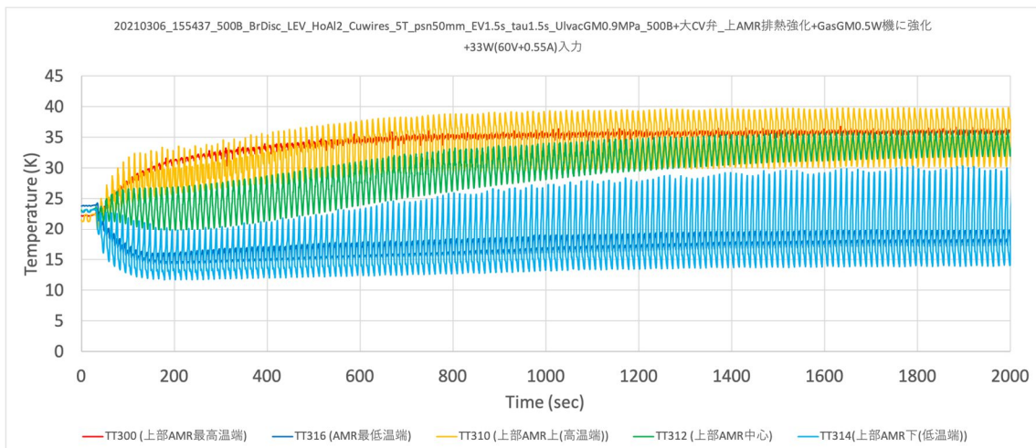
図 4 AMR 冷凍機の運転例
