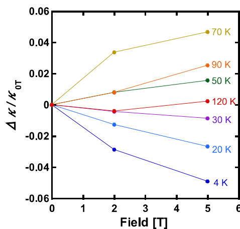
図6 GdNi_2 熱伝導率の磁場依存性
