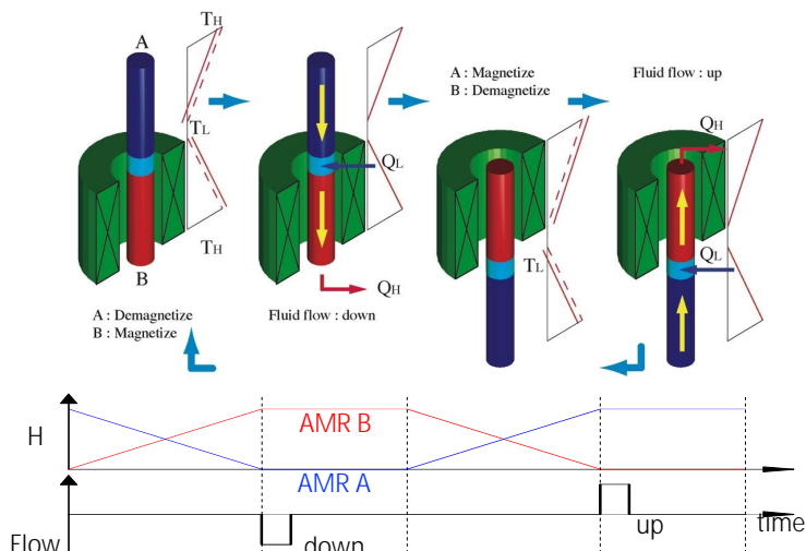
図 3 AMR 冷凍機の動作
