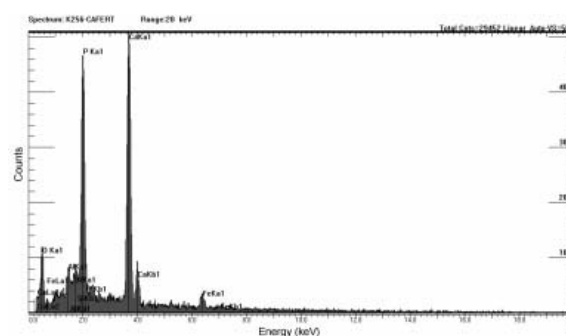
図 6 皿 ( K256 ) の SEM-EDS 分析の結果 ( 写真 25 に矢印 ↑ で示された部分 )
