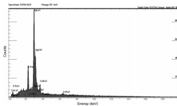
図 4 皿 ( K256 ) の SEM-EDS 分析の結果 ( 写真 24 に矢印で示された部分 )
