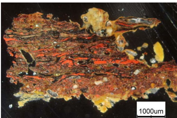
写真 35 土壌ごと包埋した塗膜断面（反射光）
