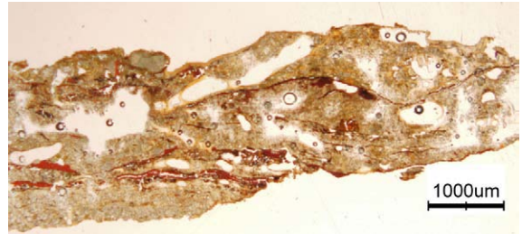
写真 30 塗膜断面（透過光）
