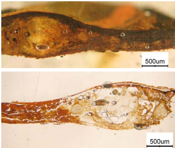
写真 14 No. 5 の断面 (上 : 反射光, 下 : 透過光)
