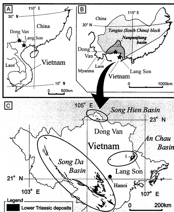
図1. A, 北部ベトナムにおける調査地域. B, 南中国ブロックに分布する下部三畳系ナンパンジャン海盆の古地理図 (Komatsu et al. , 2014 を改訂). C, アンチョウ, ソンヒエン, ソンダ堆積盆地の下部三畳系堆積物の分布. 主な調査はドンパン地域やランソン地域で実施.
