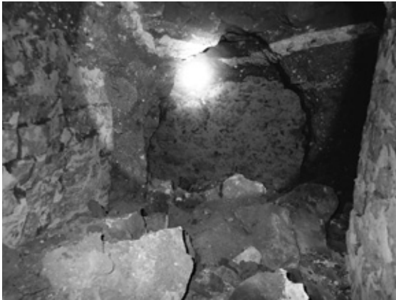
Fotografía 4. Área del colapso del túnel I-27 en Septiembre de 2017.
