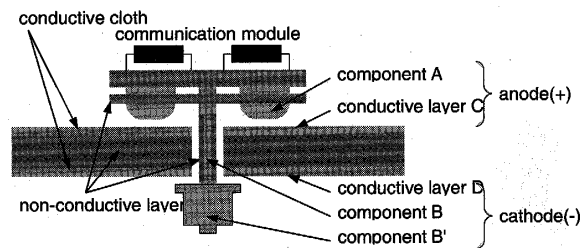
図5 ピンバッジ型インタフェース
