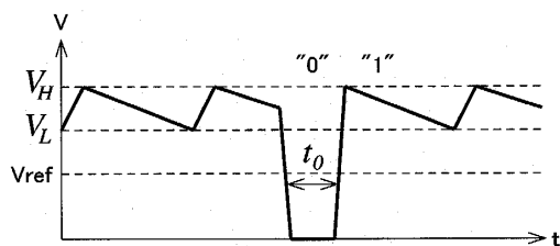
図3 TextileNet 動作時の衣服表面電圧の変化
