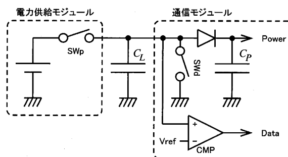
図2 TextileNet システムの等価回路
