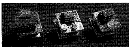
図 10 試作した衣服装着型デバイス (左から数値表示 LED デバイス, 光センサデバイス, 2色 LED デバイス)
