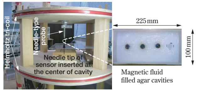
(a) 概略 (b) 励磁システムと測定サンプル 図6 磁性流体の濃度検出のための計測システム
