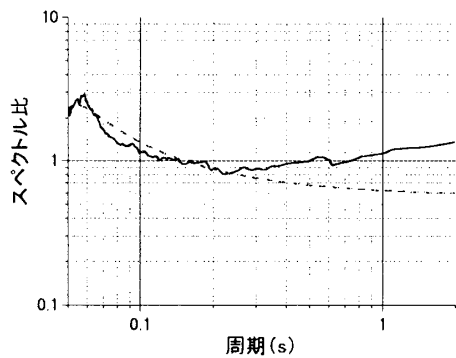
(a) 金沢大学工学部の微動 H/V とレイリー波の理論 H/V
