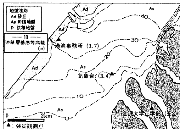
図2 金沢市の地盤図
