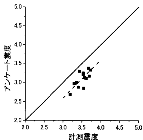
図14 アンケート収集枚数が少ない地点を除いた場合の計測震度とアンケート震度の関係
