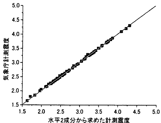
図7 水平2成分から求めた計測震度と気象庁計測震度の関係
