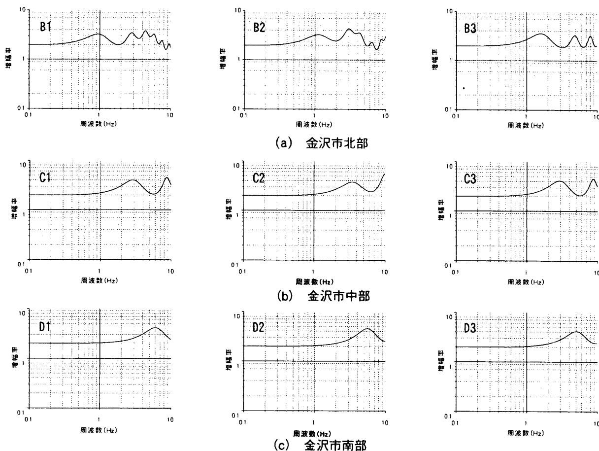
図10 地下構造より求めた増幅率
