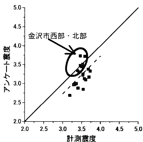
図13 計測震度とアンケート震度の関係
