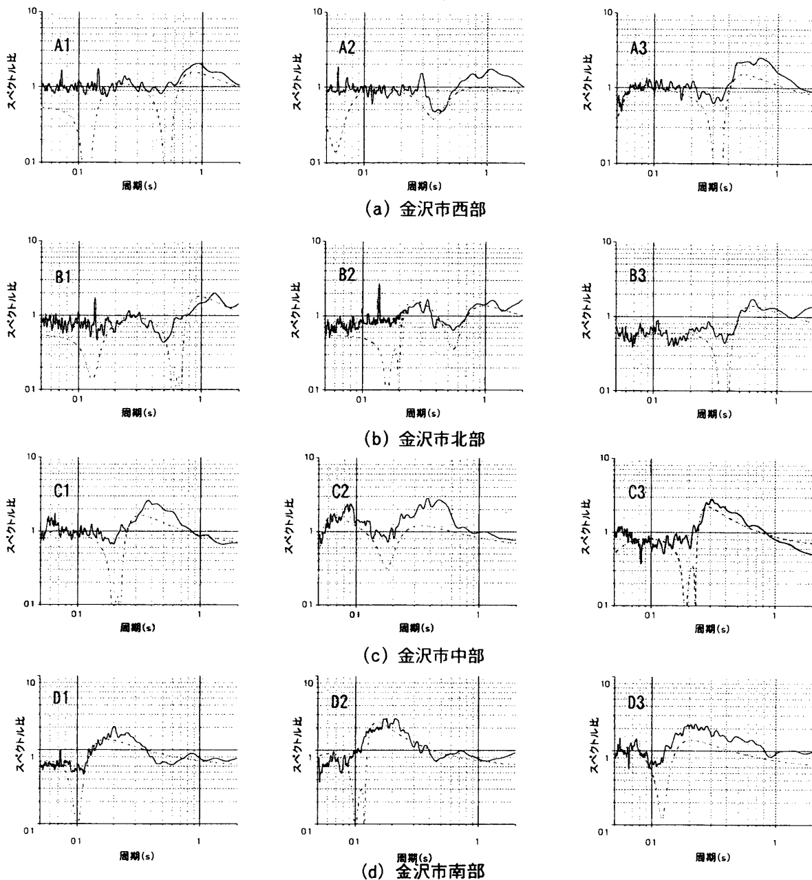
図4 微動 H/V とレイリー波の理論 H/V (実線は微動 H/V, 破線はレイリー波の理論 H/V)
