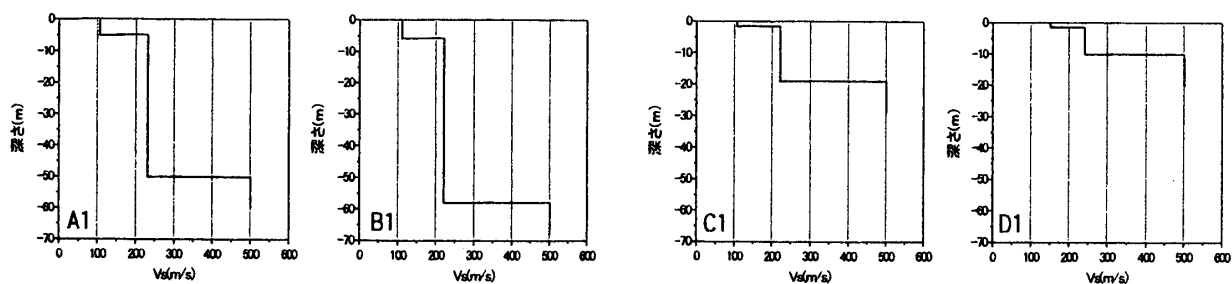
図5 逆解析より求めた地下構造
