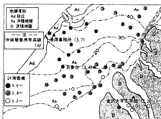
図11 地表での計測震度分布
