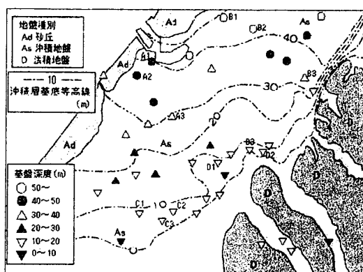
図6 金沢市の沖積層厚さと推定基盤深度分布
