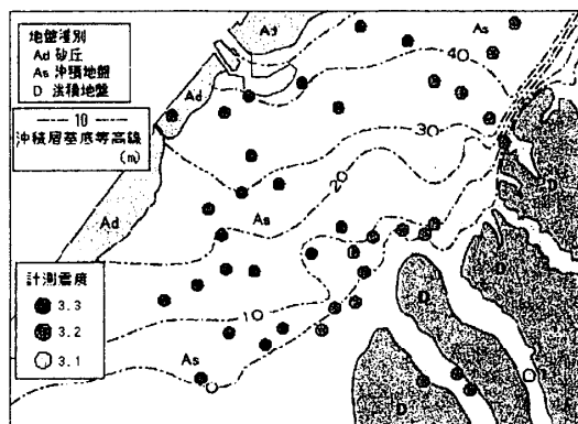
図9 工学的基盤での計測震度分布
